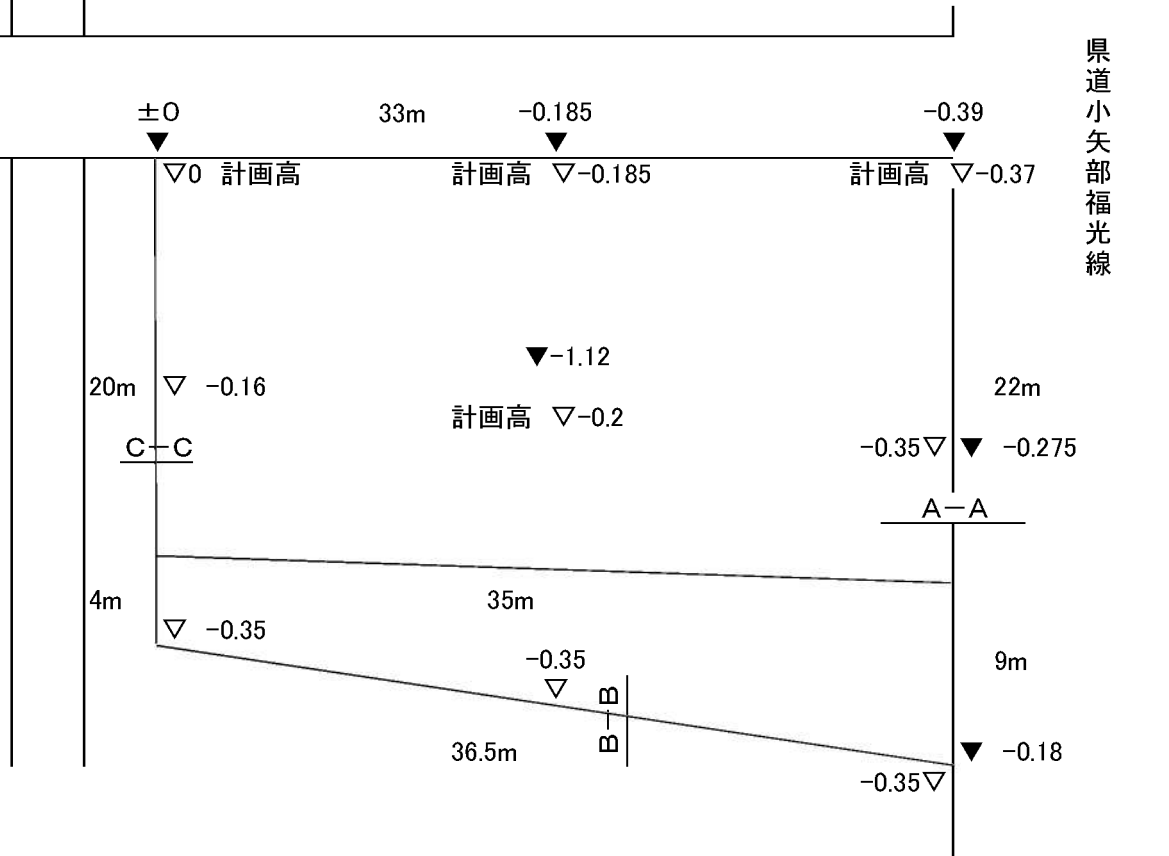
C-C断面図(略図)
