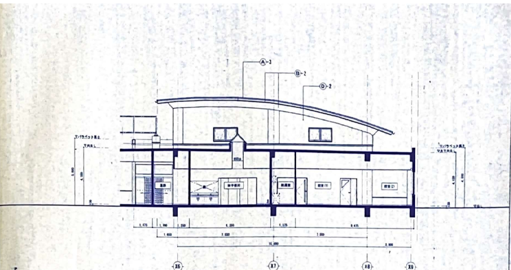
B-B' 断面図 S=1:100
