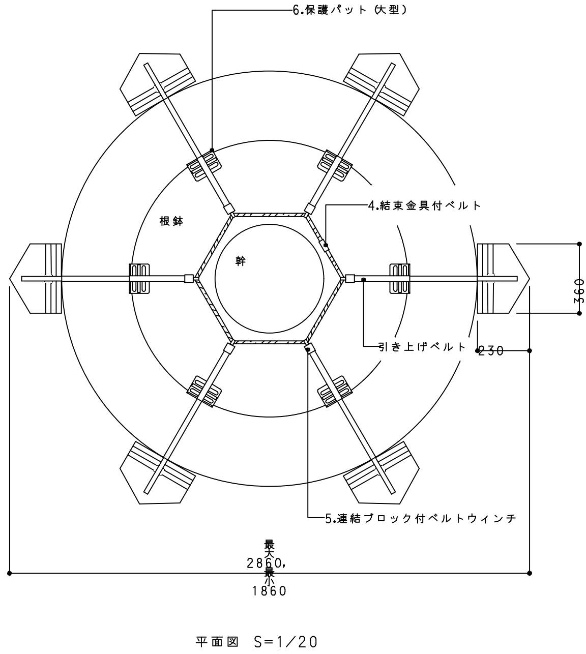
地下支柱-A（C=60 90cm）詳細図
