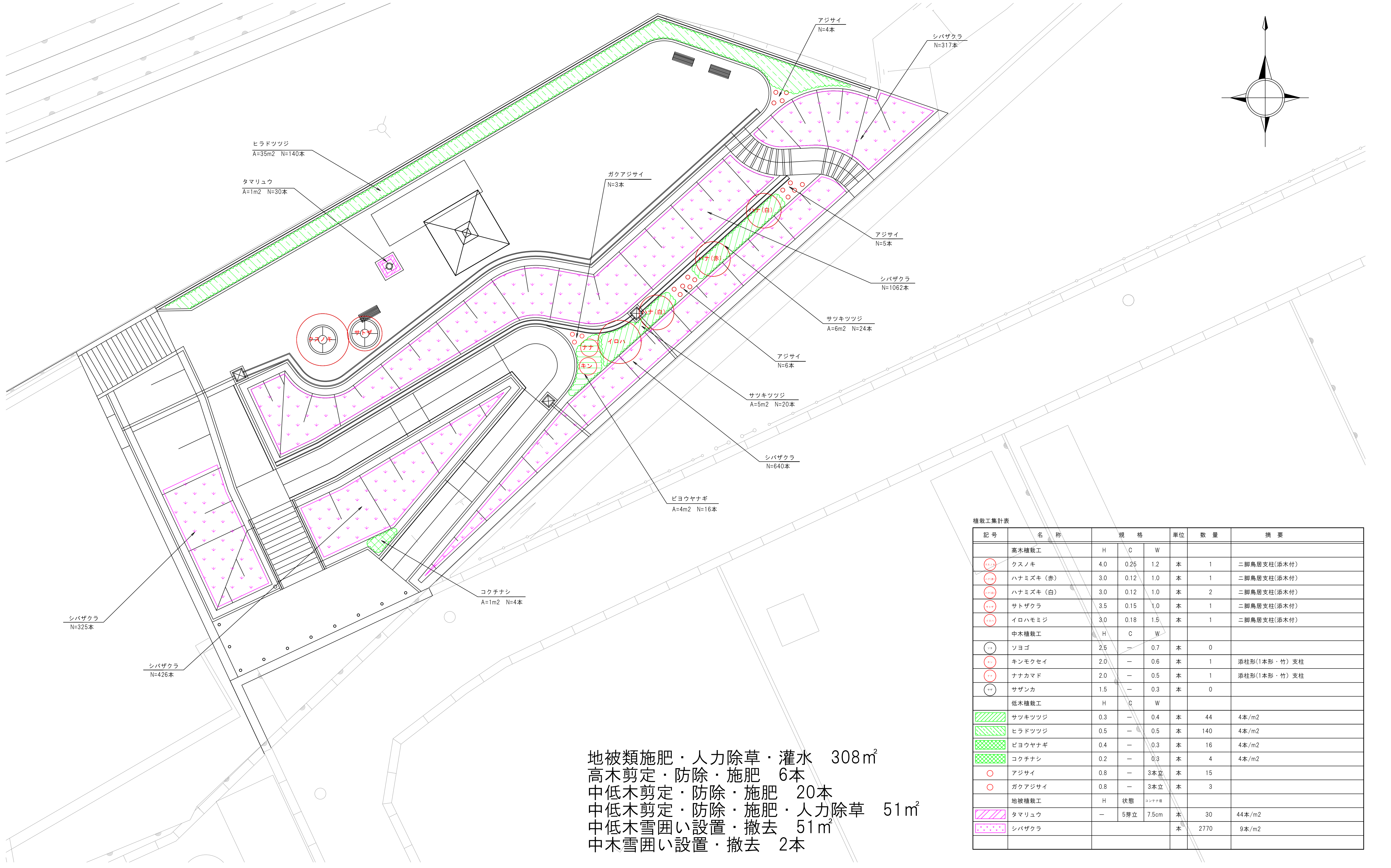
駅南口公園平面図
