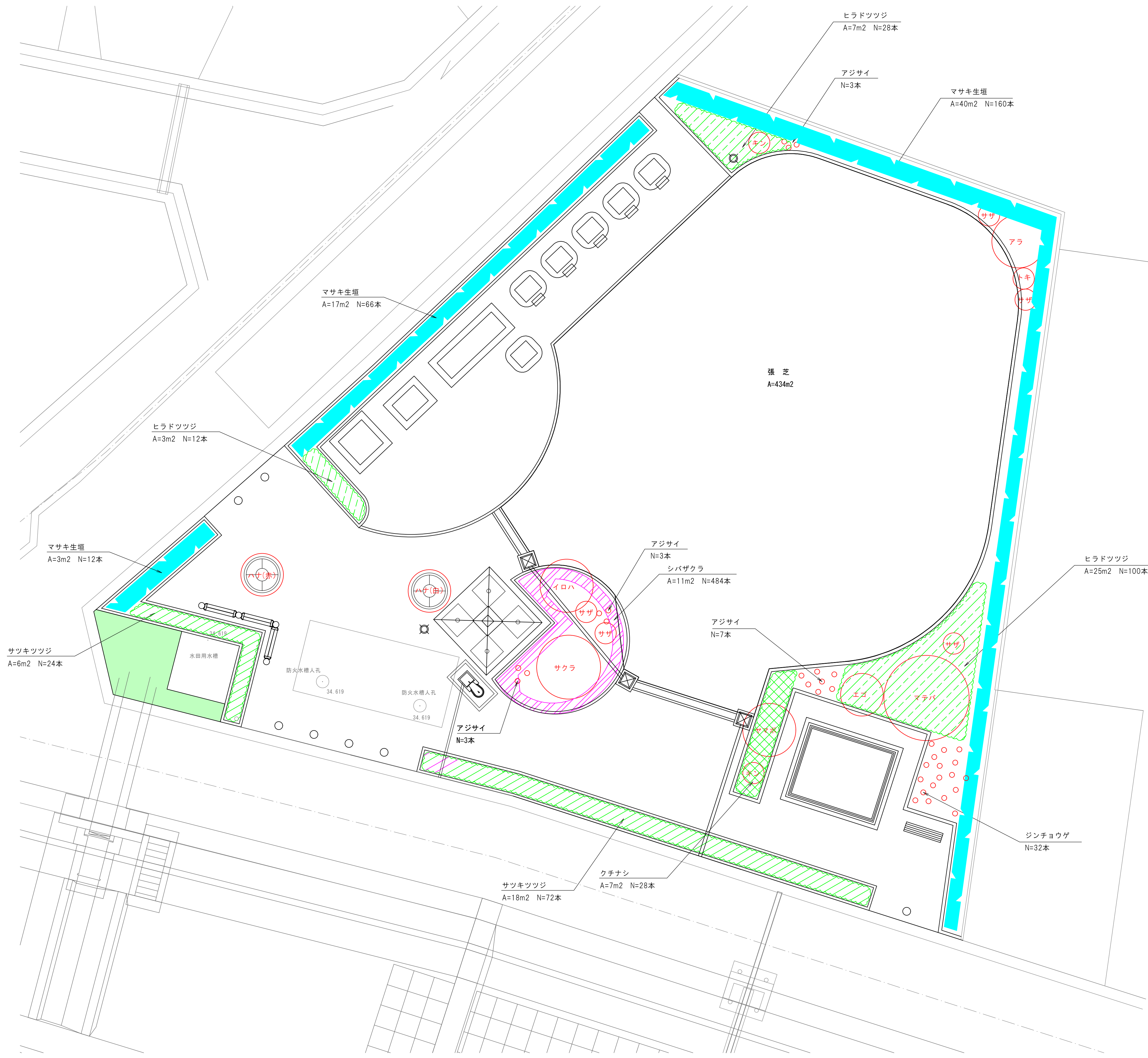
かがやき公園平面図
