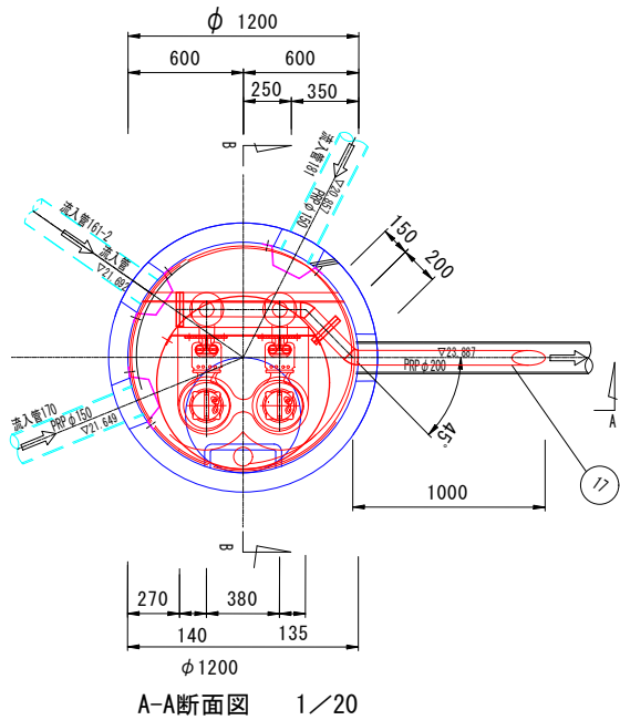
A-A断面図 1/20
