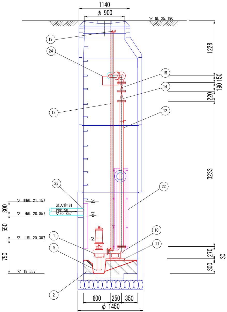
B-B断面図 1/20
