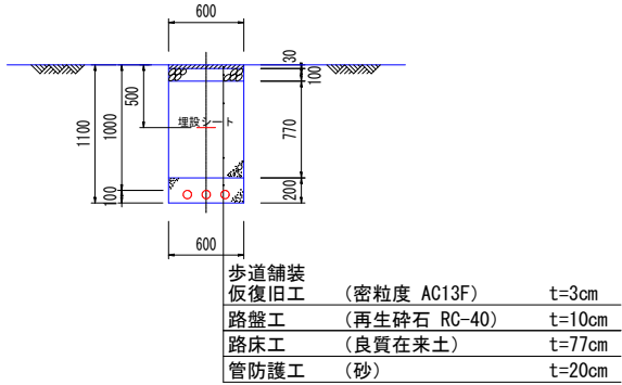
電線管布設復旧図 1/30
