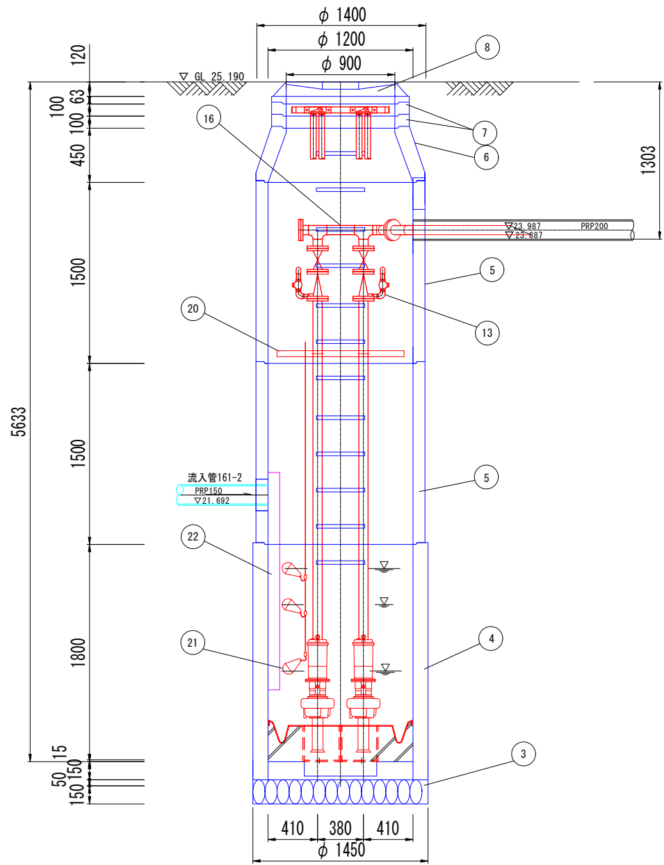
A-A断面図 1/20
