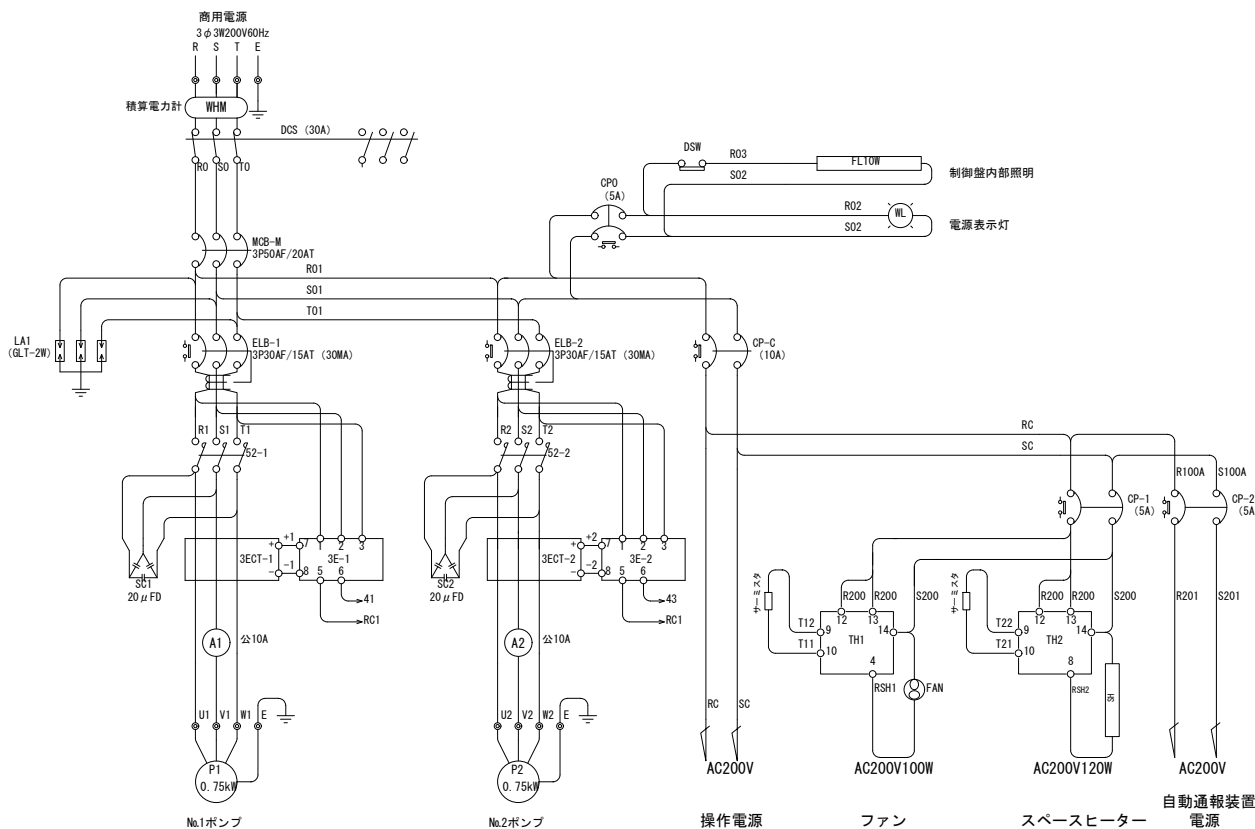
三線結線図
