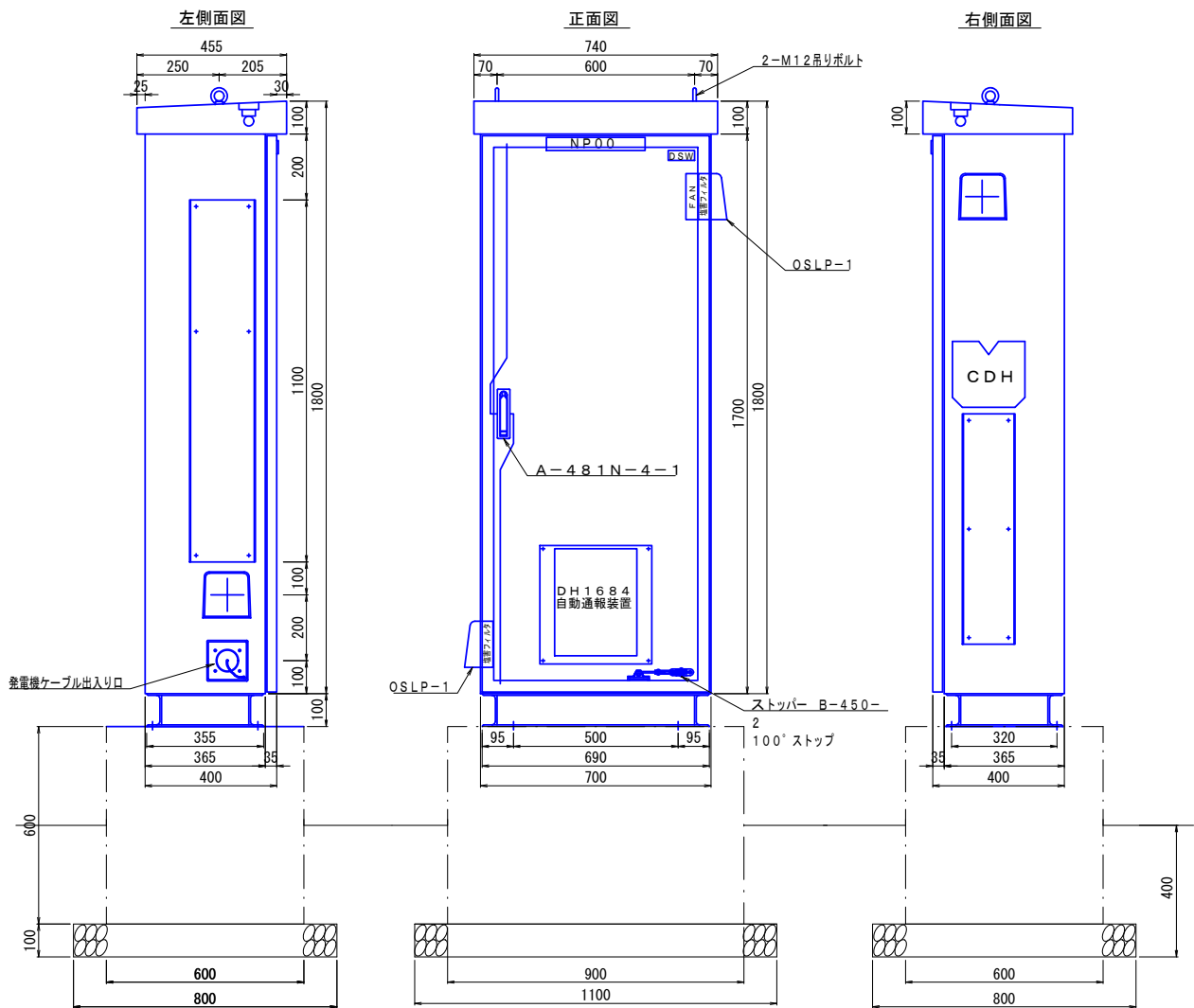
自立型操作盤外形図 S=1:10
