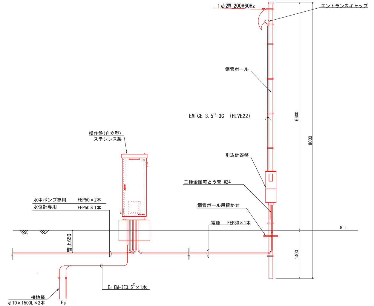
装柱図 S=1:30
