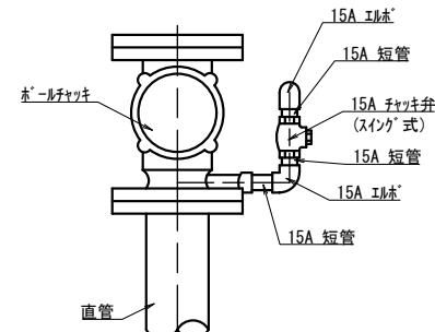
13 空気抜き配管(1式) 材質 SUS304 ネジ込み式
