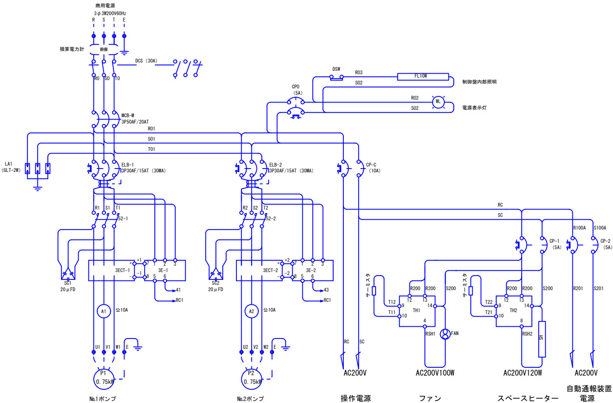
三線結線図
