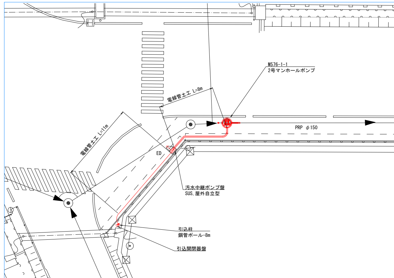
電線管布設復旧図 S=1:20
