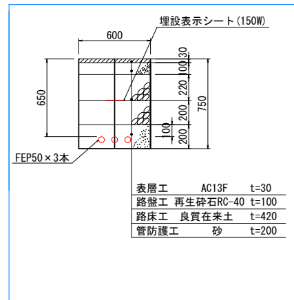
電線管布設復旧図 S=1:20
