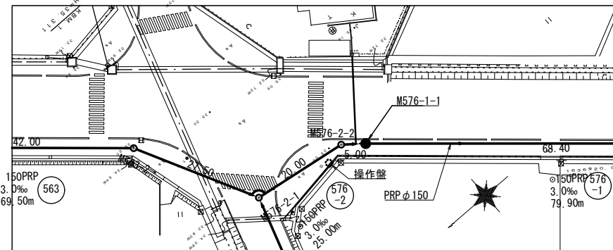
位置図 S=1:500
