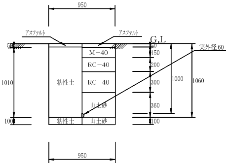
06:配水管φ50 01: HPPEφ50 H=1000(L) 下水同時 (掘削・埋戻し)
