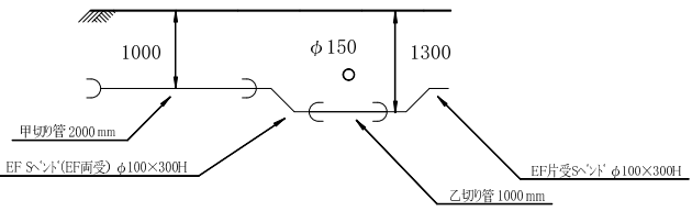
A部詳細図
