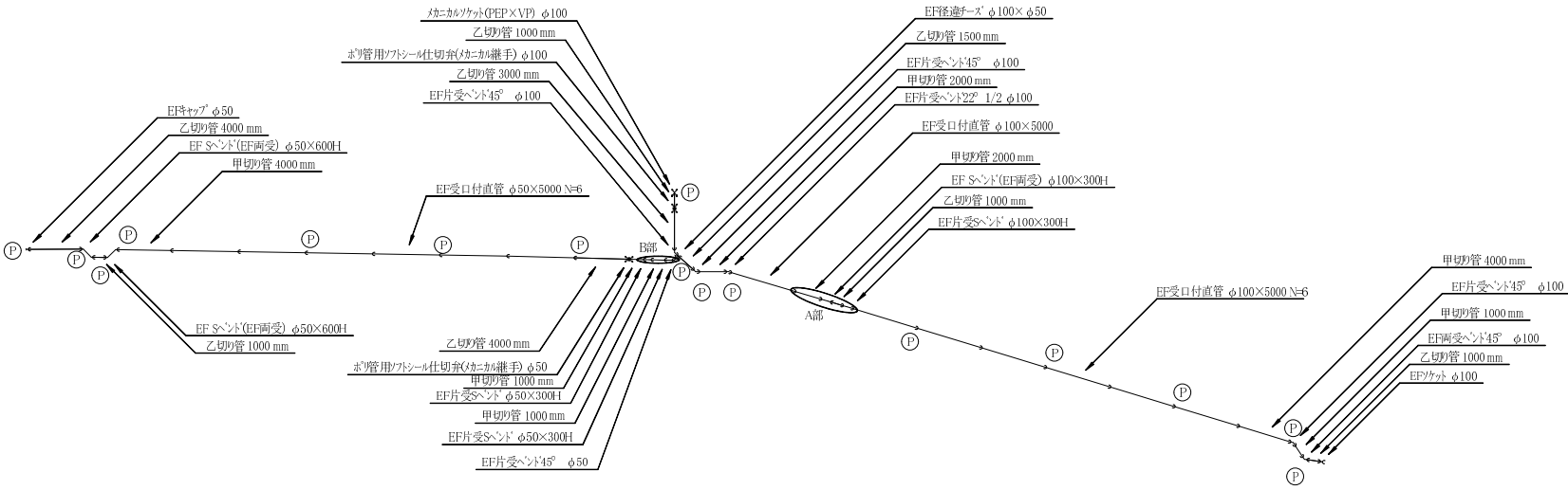
平面詳細図 S=1/250
