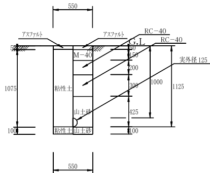
00:配水管φ100 02: HPPEφ100 H=1000(L) 単独 (掘削・埋戻し)
