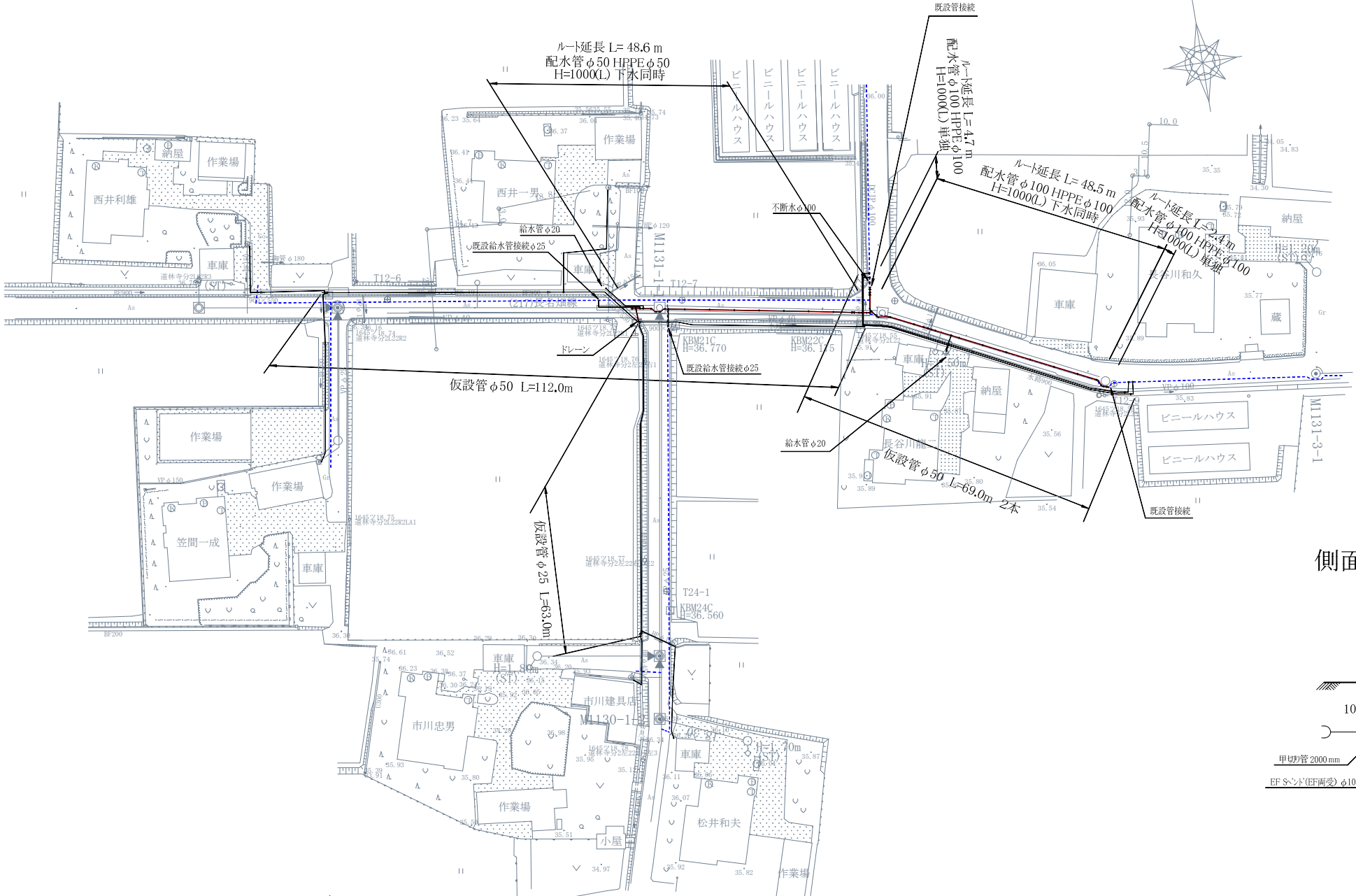
平面詳細図 S=1/250
