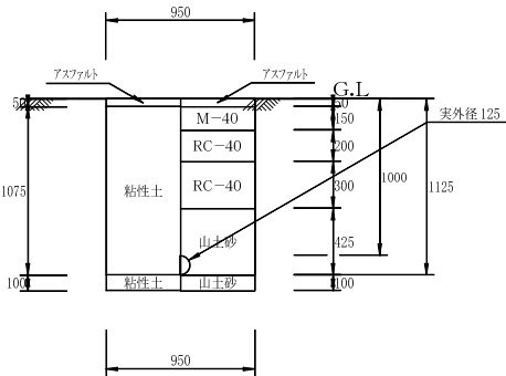
00:配水管φ100 01: HPPEφ100 H=1000(L) 下水同時 (掘削・埋戻し)
