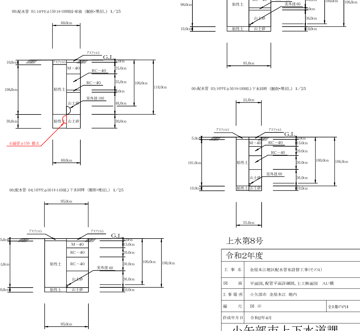
土工断面図 S=1/25
