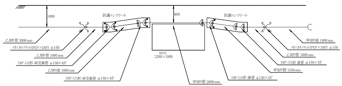
A部詳細図 S=1/50
