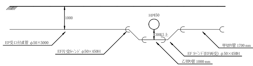
B部詳細図 S=1/50
