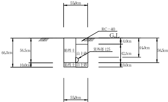
00:配水管 03: HPPEφ100 H=440 単独(掘削・埋戻し)
