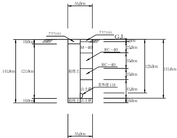
00:配水管 09: DIPGXφ100(B) L=1200 単独(掘削・埋戻し)
