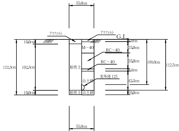
00:配水管 01: HPPEφ100(B) H=1000 単独(掘削・埋戻し)
