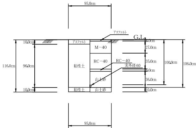
00:配水管 10: HPPEφ50 下水同時 (掘削・埋戻し)
