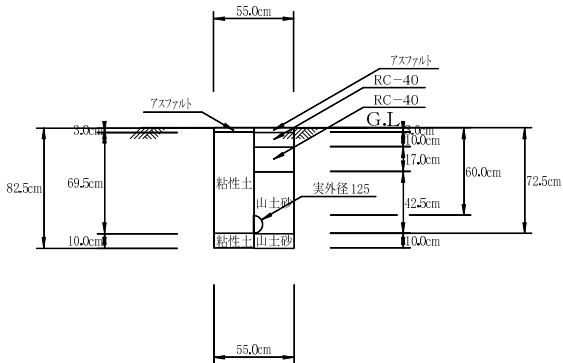
00:配水管 05: HPPEφ100(歩道)H=600 単独(掘削・埋戻し)
