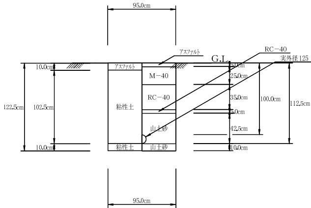
00:配水管 02: HPPEφ100(B) H=1000 下水同時 (掘削・埋戻し)
