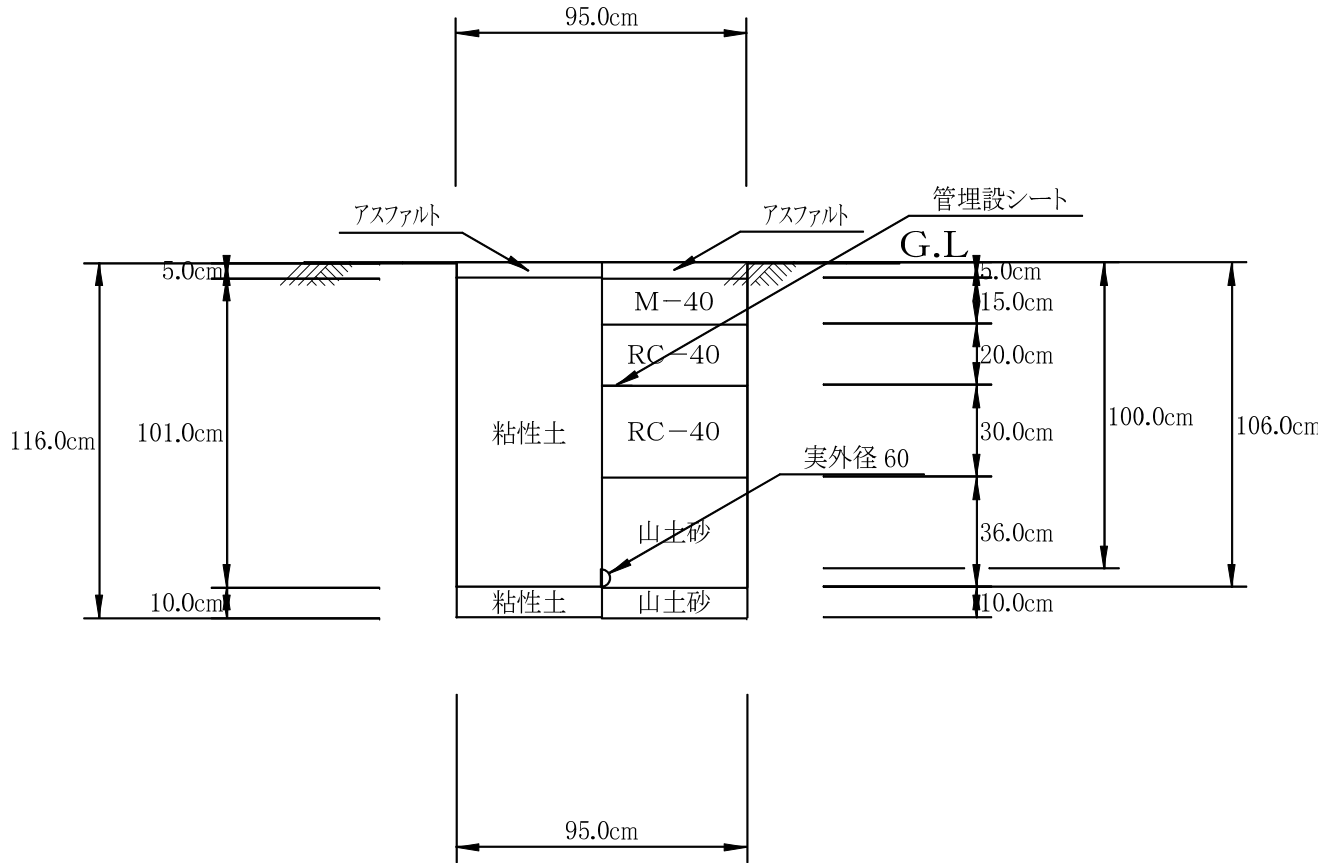
00:配水管 02: HPPE φ50下水同時（掘削・埋戻し） 1／25
