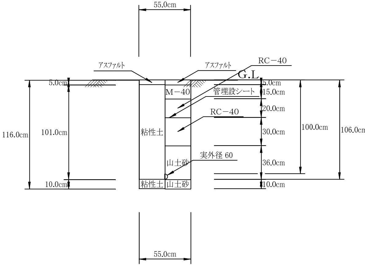
00:配水管 01: HPPE φ50上水単独（掘削・埋戻し） 1／25
