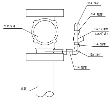
B-B断面図 1/20
