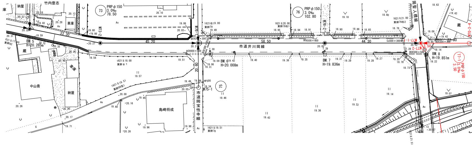
平面図 縮尺1:500
