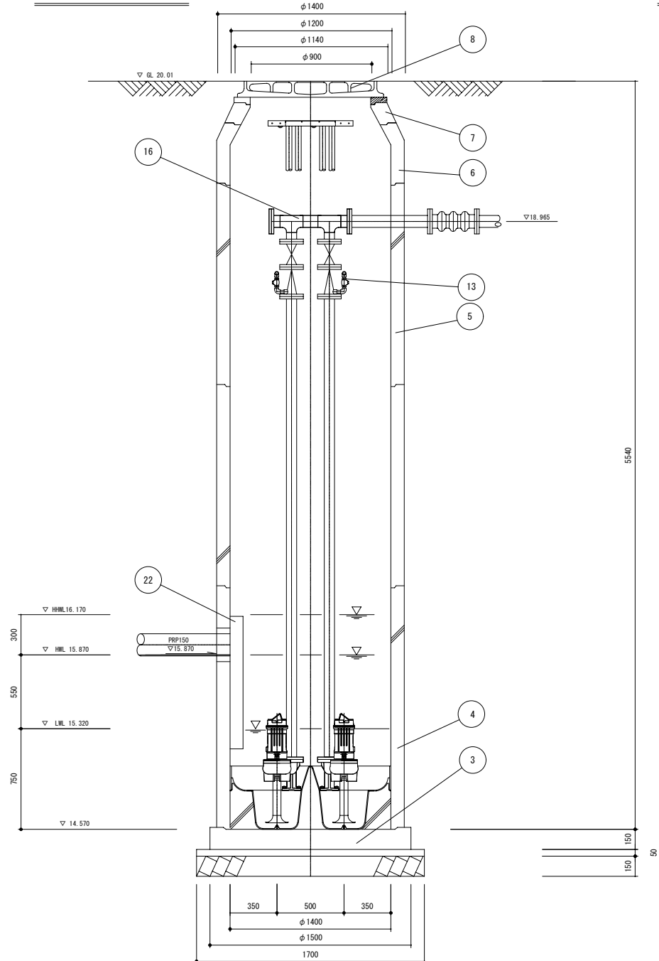
A-A断面図 1/20
