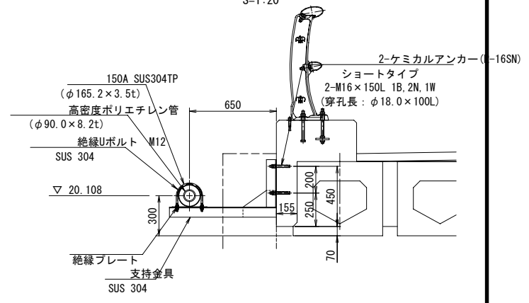
断面図 S=1:20
