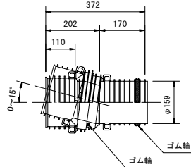
自在継手 150
