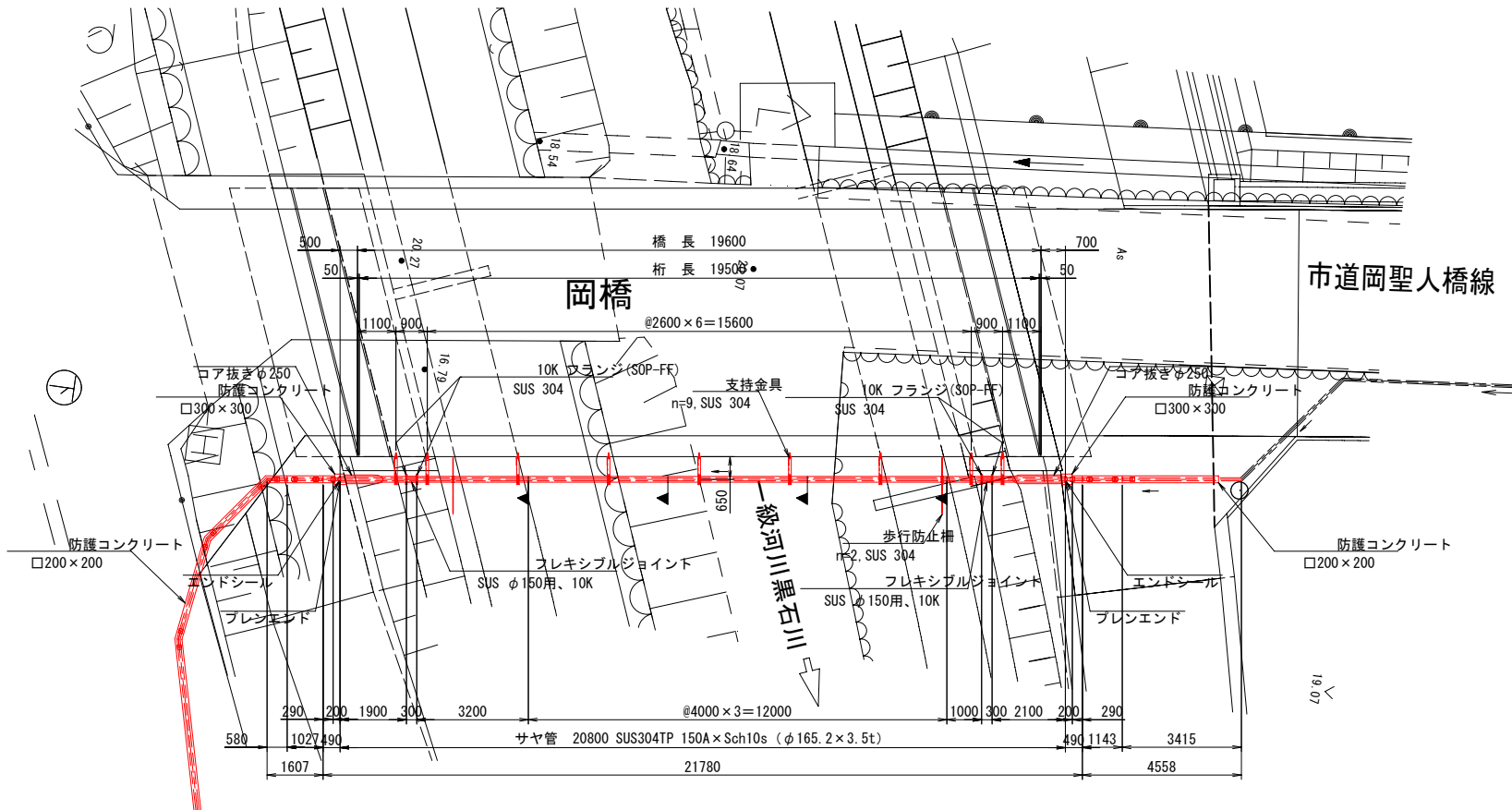
平面図 S=1:100
