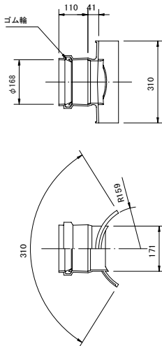
マルチ支管 300-150
