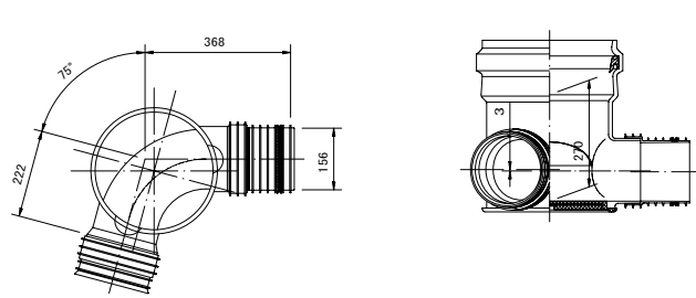
曲点インバート 75° 曲り
