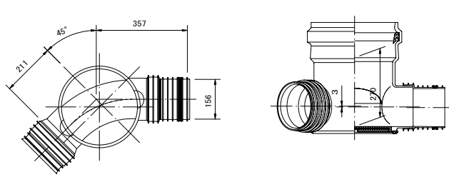
曲点インバート 45° 曲り
