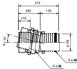
自在継手 150
