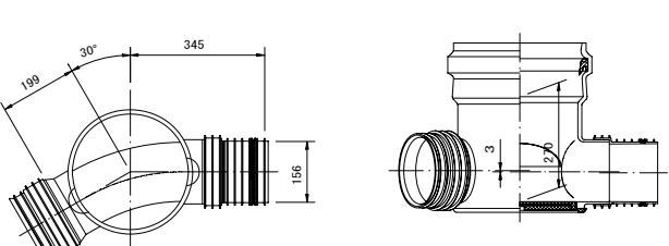
曲点インバート 30° 曲り
