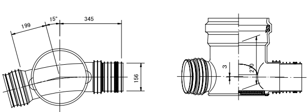
曲点インバート 15° 曲り
