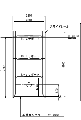
B-B' 断面図
