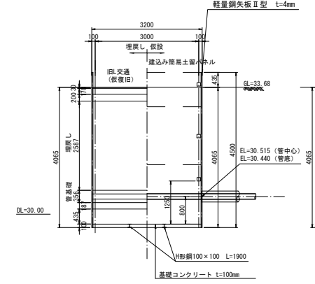
A-A' 断面図
