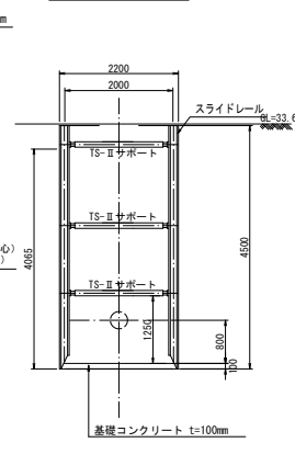
B-B' 断面図
