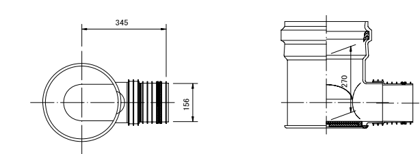
起点インバート
