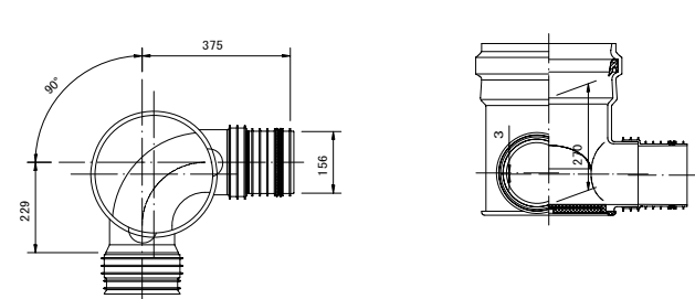
曲点インバート 90° 曲り
