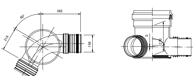
曲点インバート 60° 曲り
