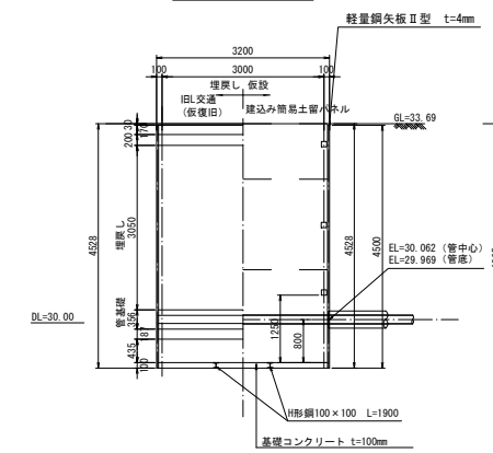
A-A' 断面図
