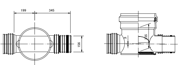
中間点インバート
