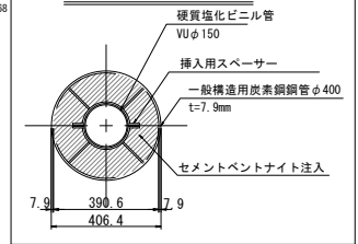
管断面図 S=1/10
