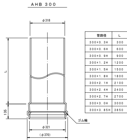
立 管
