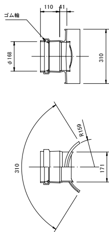
マルチ支管 300-150
