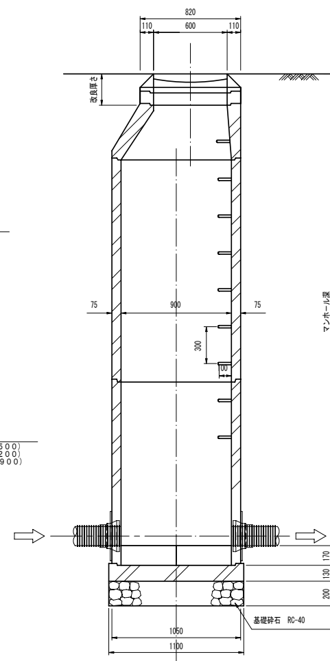
B-B' 断面图
