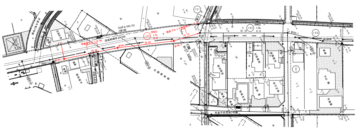
平面図 縮尺 1:1,000
