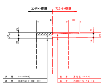
歩道部・歩道乗入部
