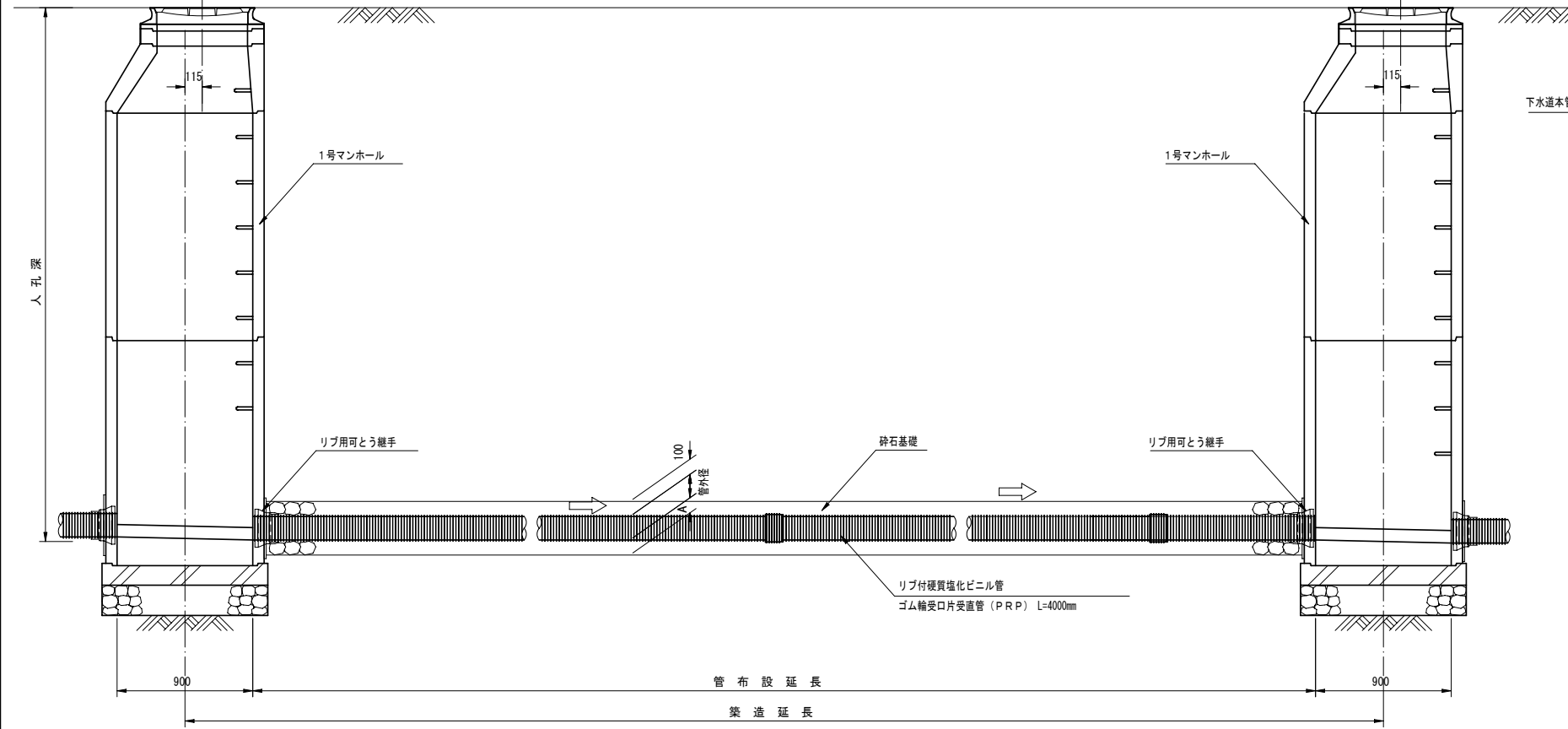
リブ付硬質塩化ビニル管寸法図
