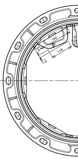
② フレーム平面図
