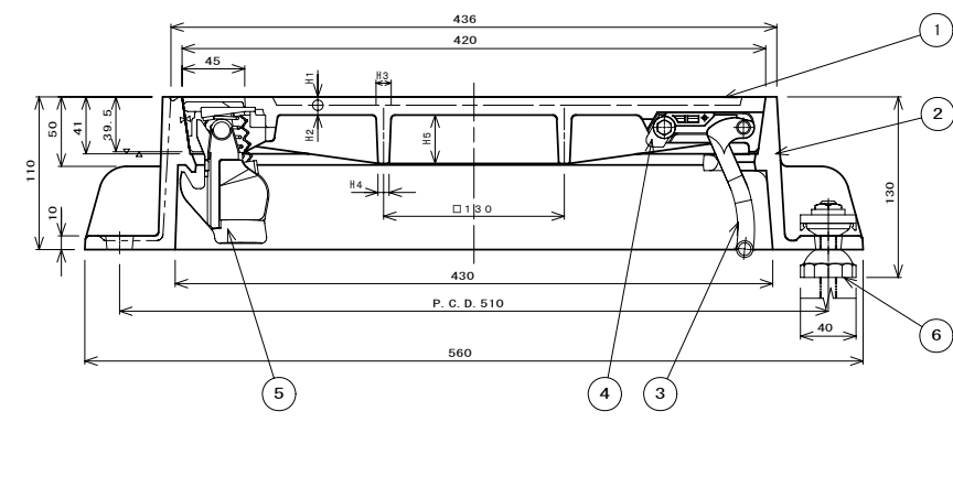
カバー、フレイム断面図
