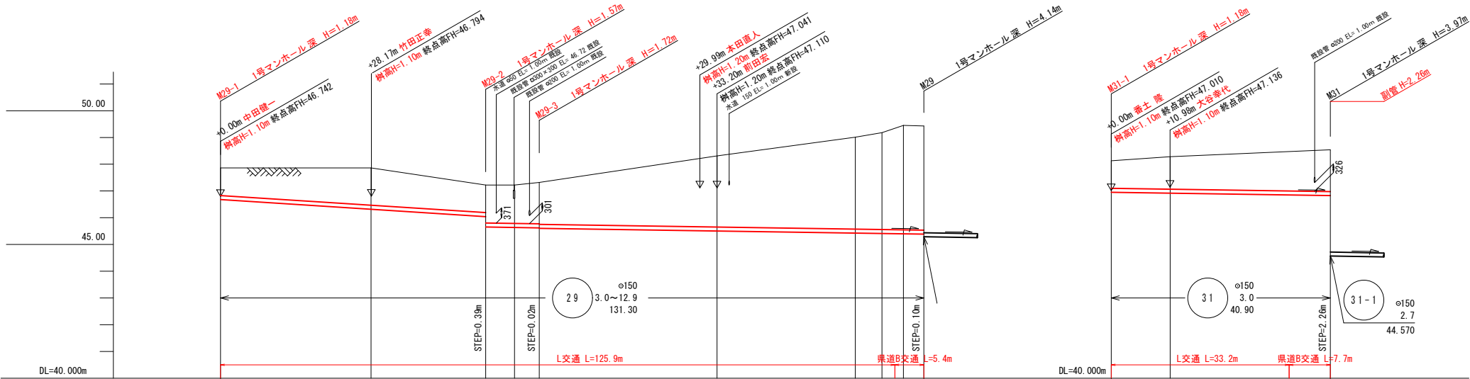
縦断面図 縦縮尺S=1:100 横縮尺S=1:500
