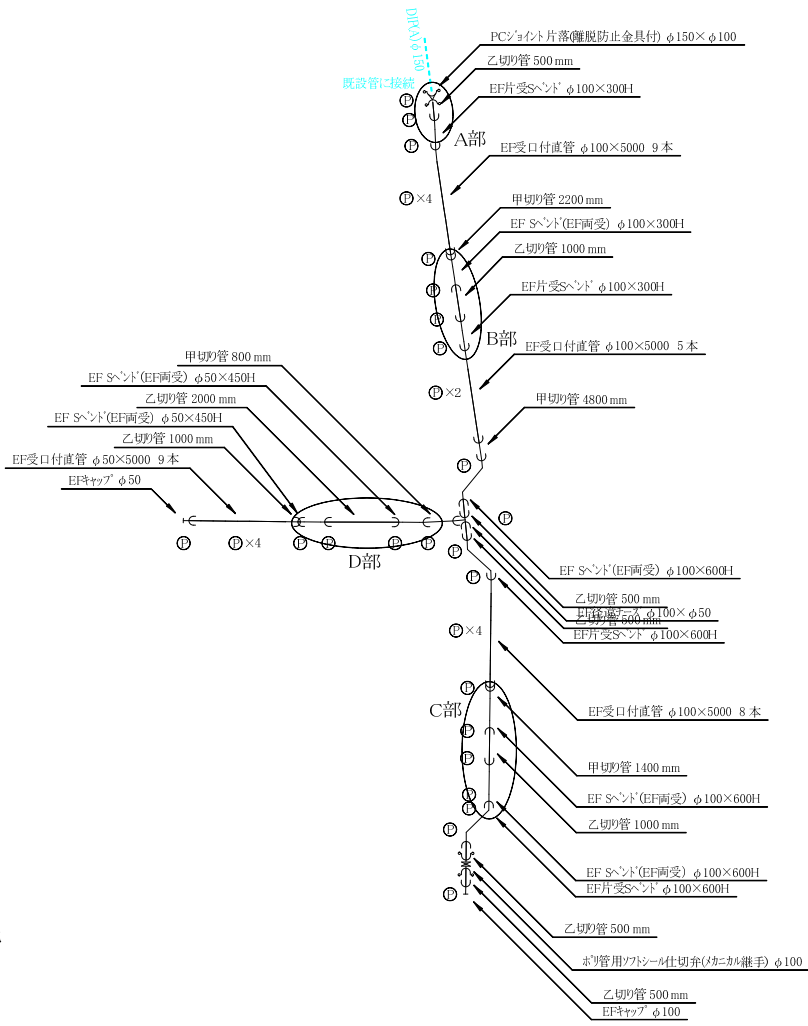
配管平面詳細図 S=1/100
