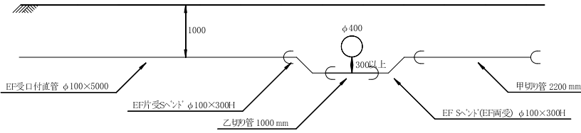
D部詳細図 S=1/50
