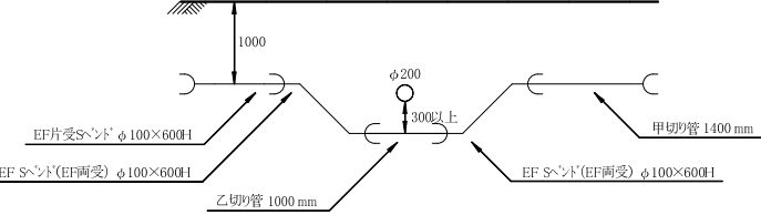
C部詳細図 S=1/50
