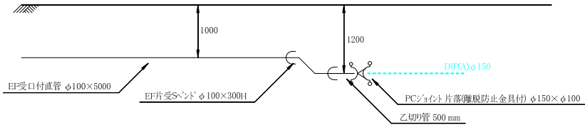
A部詳細図 S=1/50
