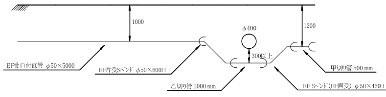
A部詳細図 S=1/50
