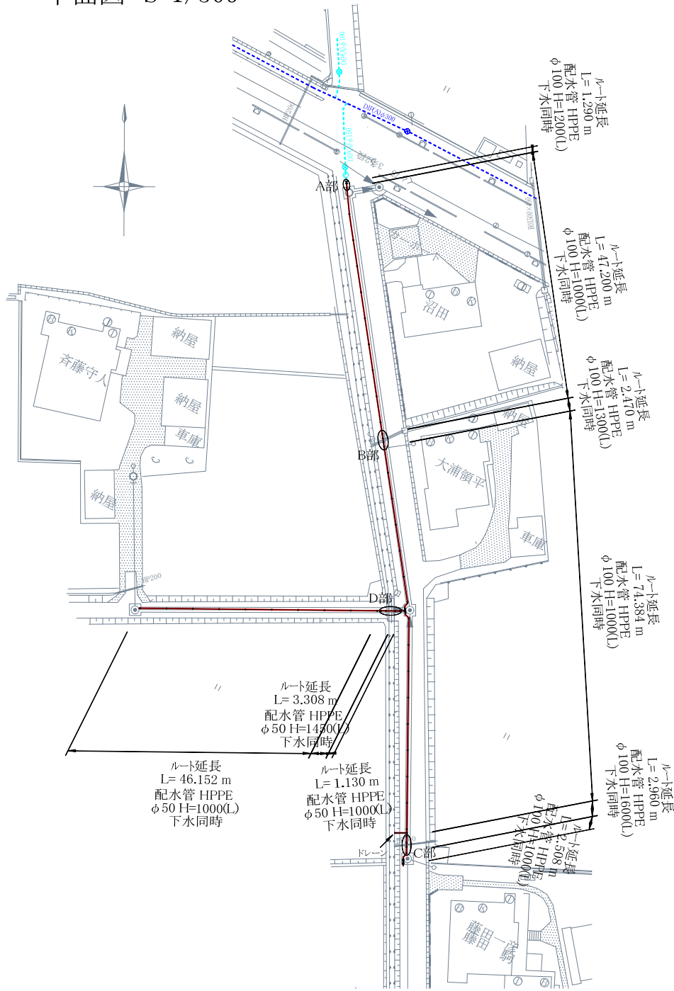
平面図 S=1/500
