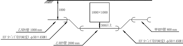
D部詳細図 S=1/50
