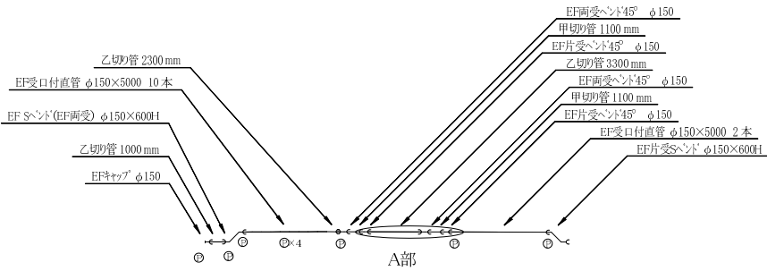
平面詳細図 S=1/200
