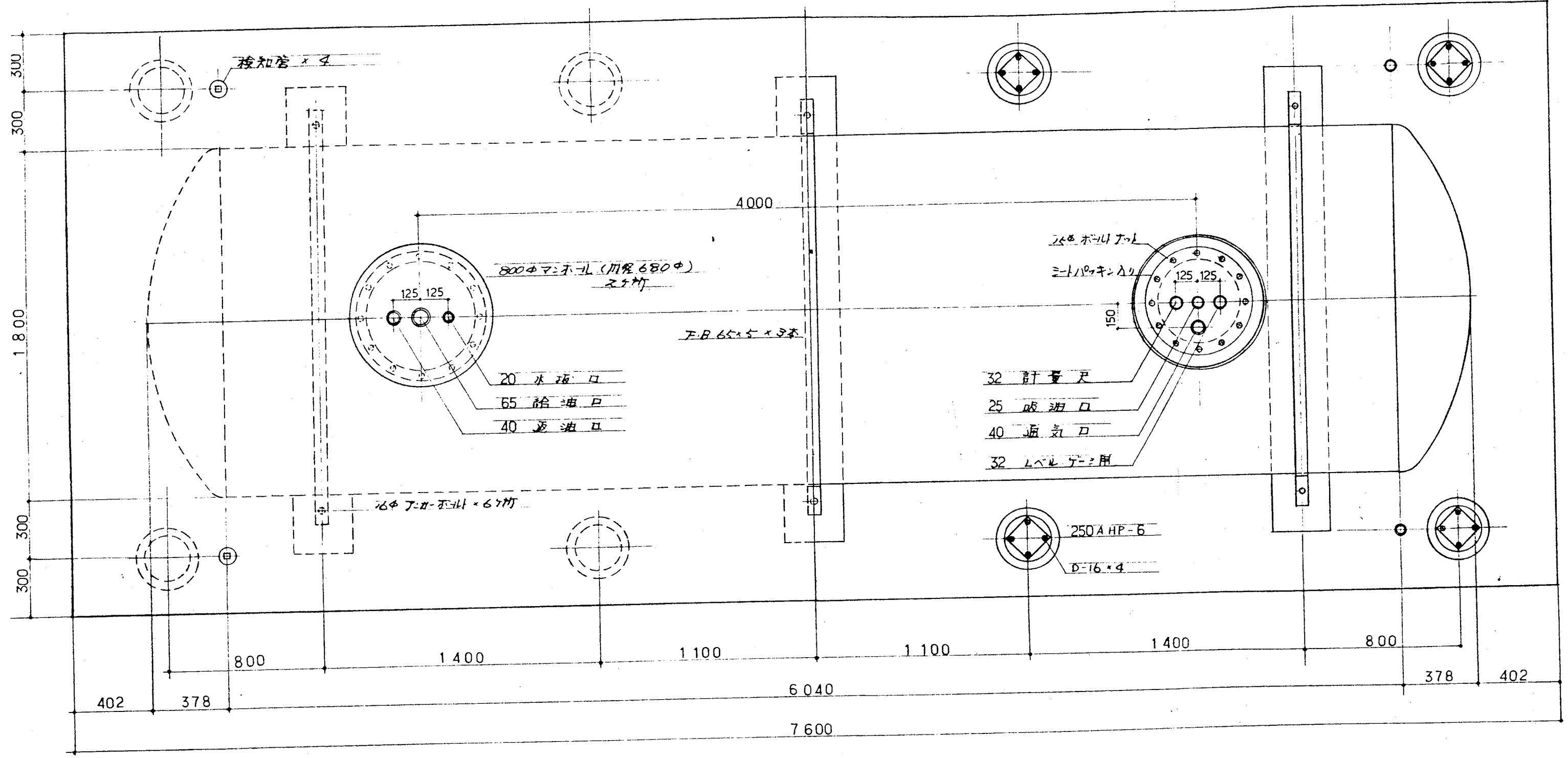
平面図
