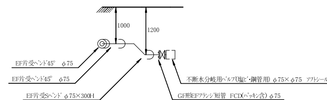
G部詳細図 S=1/50
