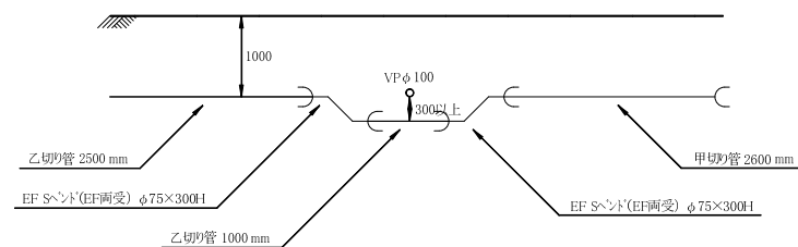
C部詳細図 S=1/50
