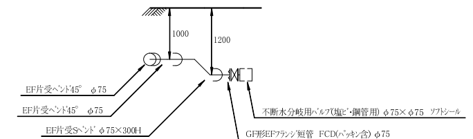
F部詳細図 S=1/50
