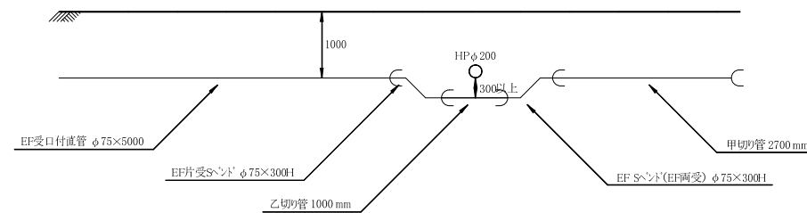
E部詳細図 S=1/50
