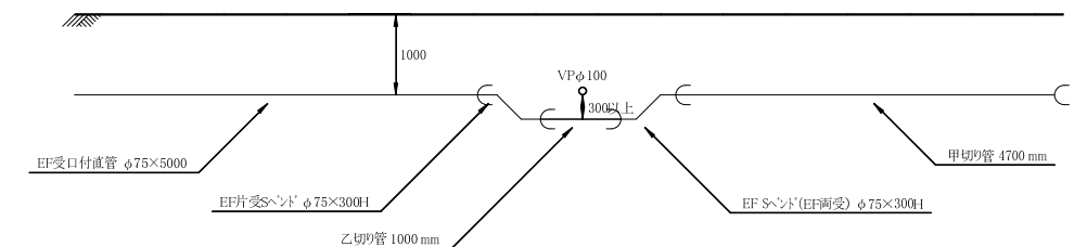
B部詳細図 S=1/50
