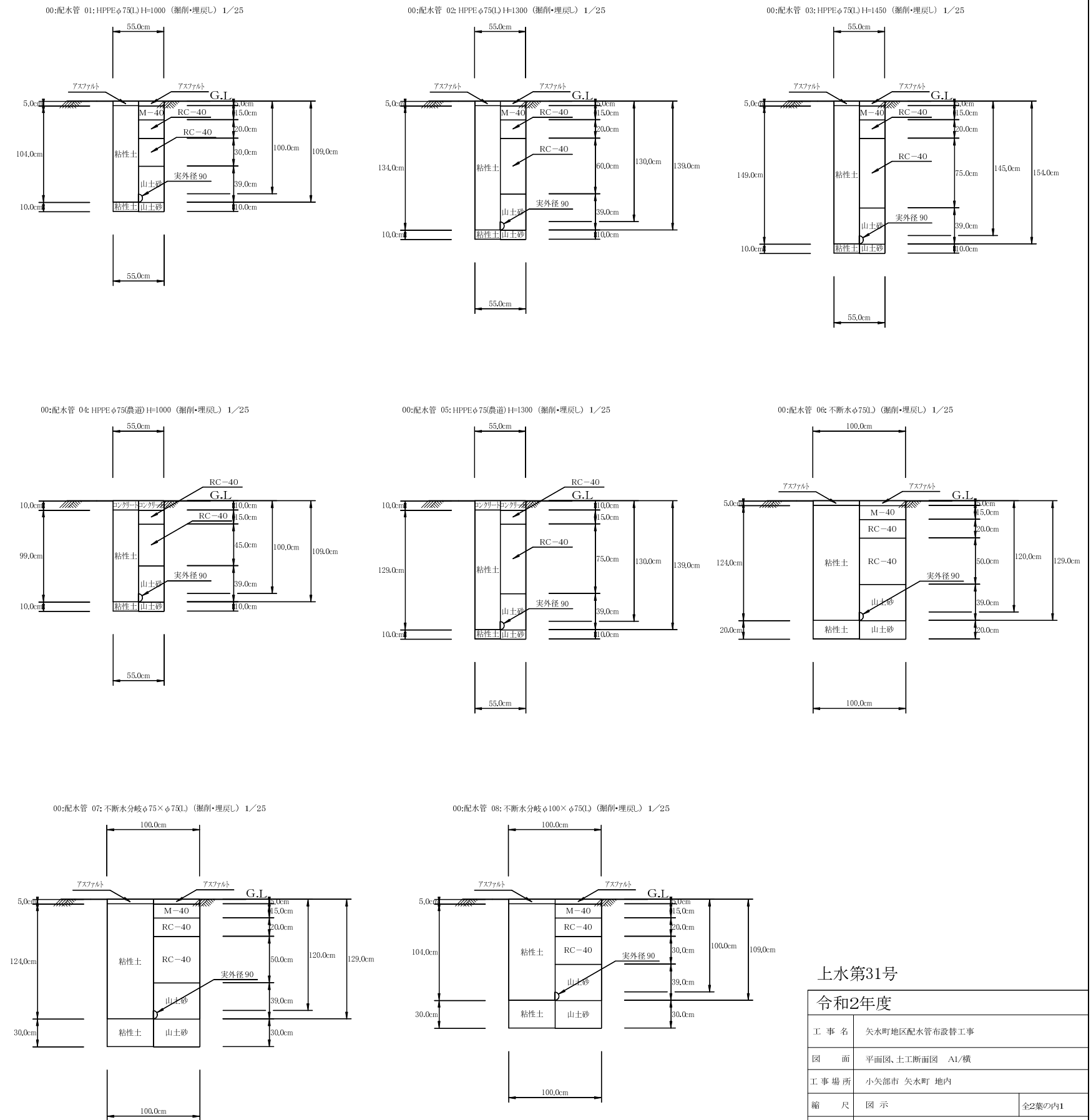
土工断面図 S=1/25
