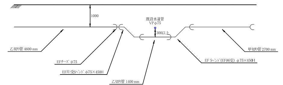
D部詳細図 S=1/50
