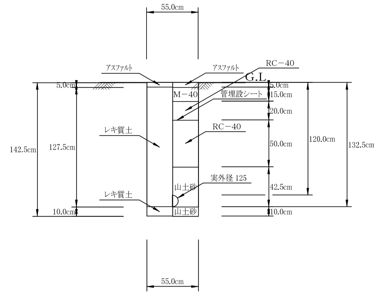
00:配水管 05: HPPE φ100上水単独(L)(H=1200) (掘削・埋戻し) 1/25
