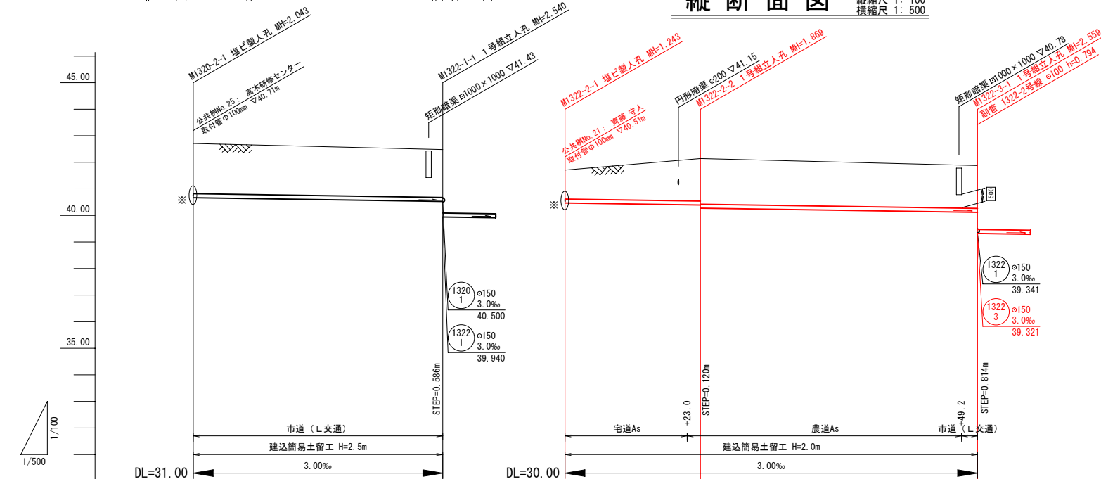
縦断面図 縦縮尺 1: 100 横縮尺 1: 500
