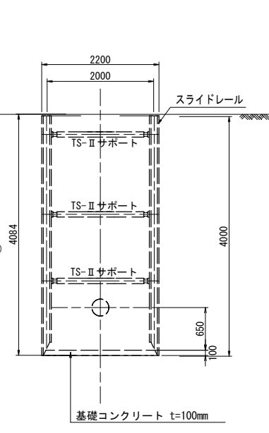
B-B' 断面図
