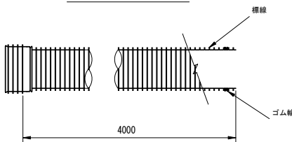
リブ付硬質塩化ビニル管寸法図
