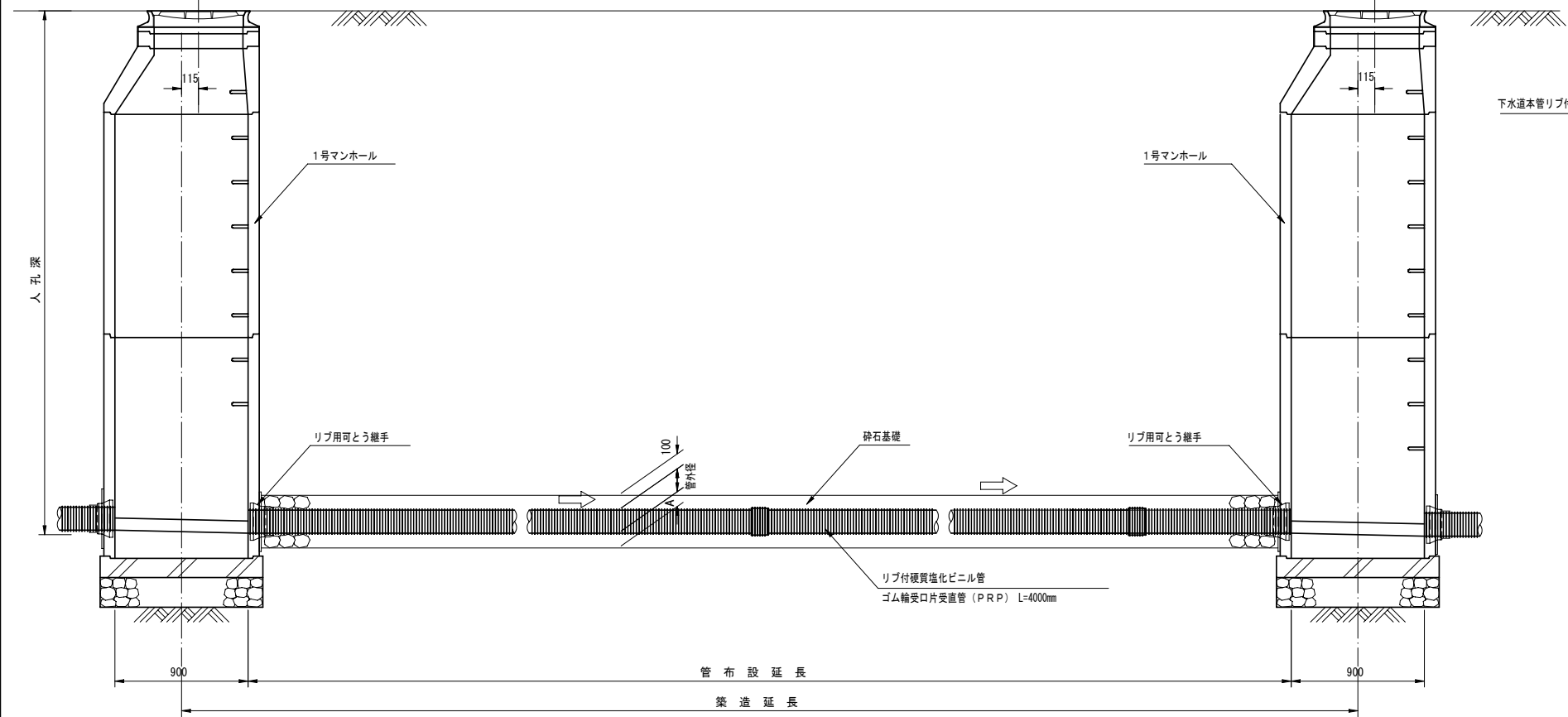
リブ付硬質塩化ビニル管寸法図
