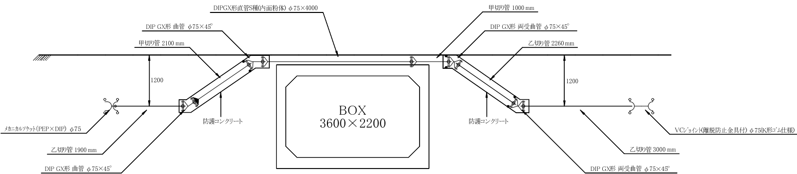
A部側面詳細図 S=1/50
