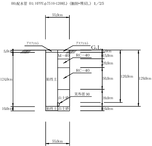
土工断面図 S=1/25
