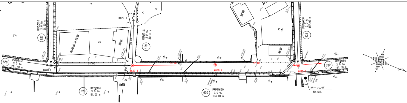
平面図 縮尺1:1,000
