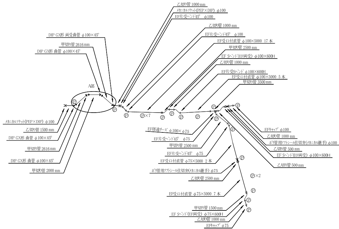
配管平面詳細図 S=1/200
