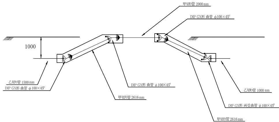
A部詳細図 S=1/50
