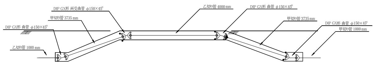
A 部 側 面 詳 細 図 S=1/50
