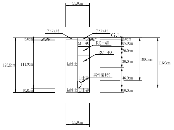
00:配水管 09: DIPGX φ150(L) H=1000 単独 (掘削・埋戻し)
