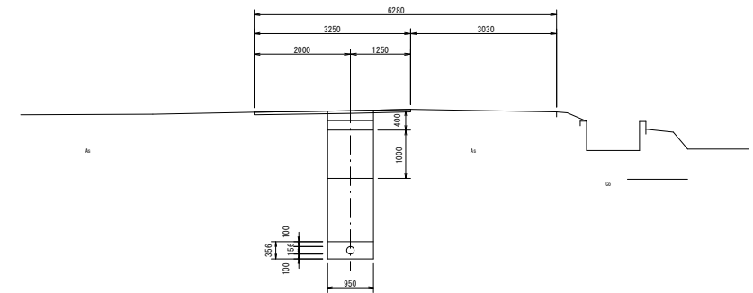
M627-1 (農道As)
