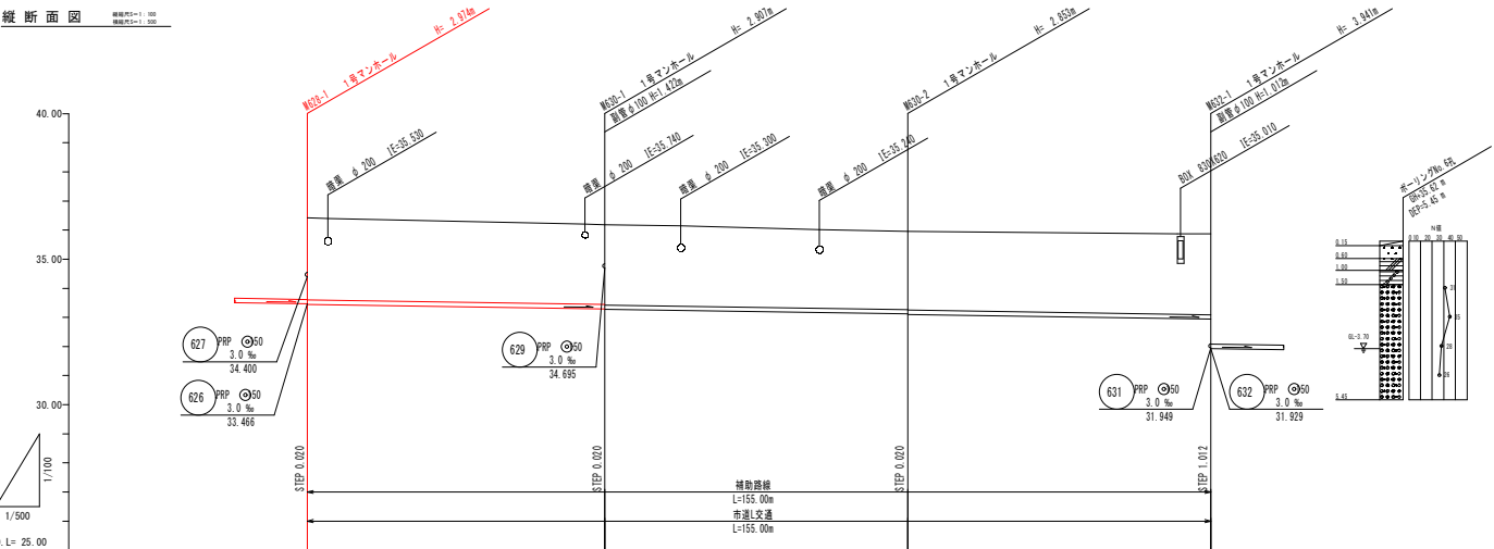
縦断面図
