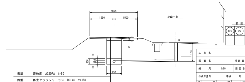
M627-1 (農道As)
