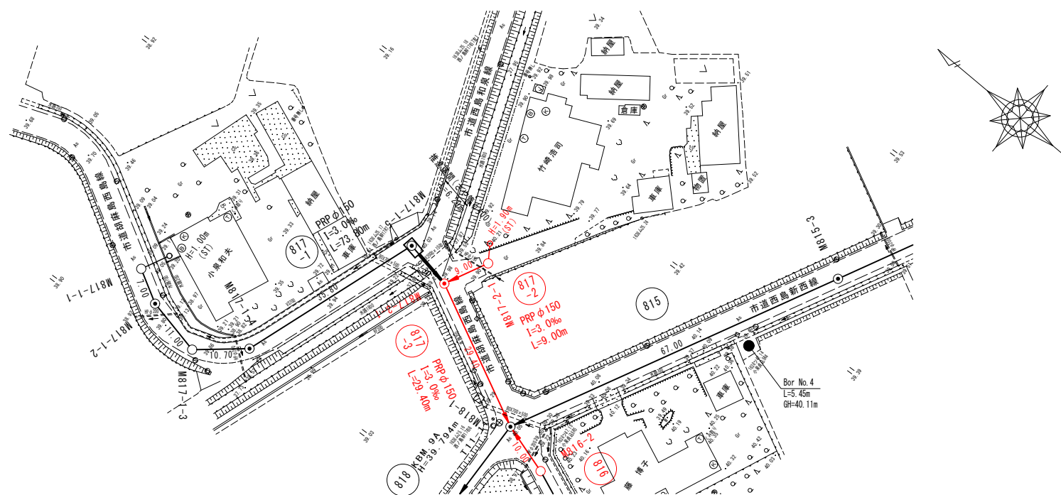
縦断面図 Sv=1:100, Sh=1:500
