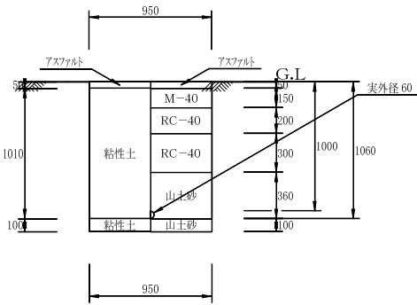
00:配水管 05: HPPEφ50 H=1000(L) 下水同時 (掘削・埋戻し)
