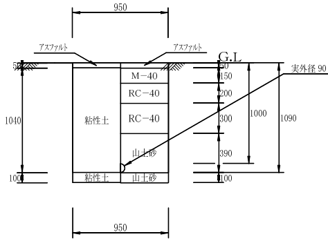
00:配水管 06: HPPEφ75 H=1000(L) 下水同時 (掘削・埋戻し)
