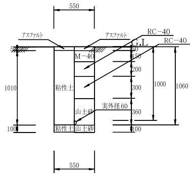
00:配水管 04: HPPEφ50 H=1000(L) 単独 (掘削・埋戻し)
