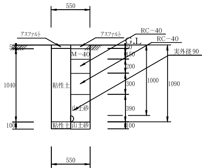
00:配水管 03: HPPEφ75 H=1000(L) 単独 (掘削・埋戻し)
