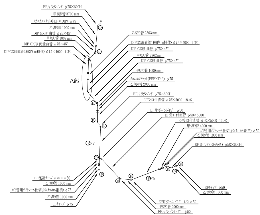
平面詳細図 S=1/200
