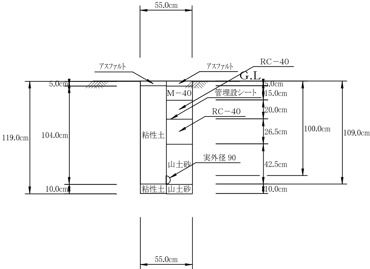
00:配水管 06: HPPE φ 75上水単独 (L) (H=1000) (掘削・埋戻し) 1／25
