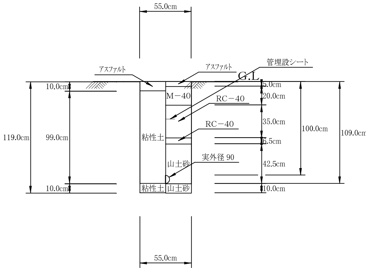
00:配水管 08: HPPE φ 75上水単独 (B) (H=1000) (掘削・埋戻し) 1／25
