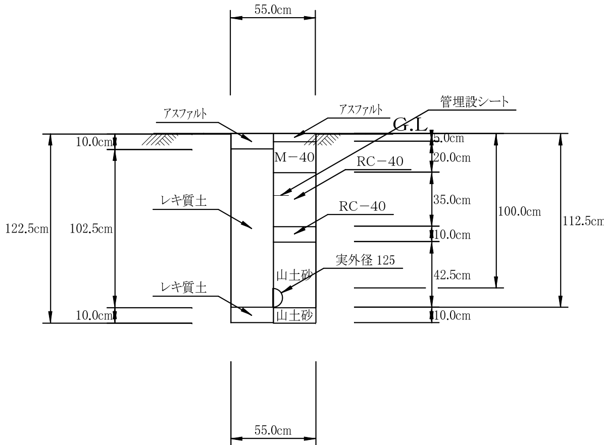
00:配水管 09: HPPE φ 100上水単独 (B) (H=1000) (掘削・埋戻し) 1／25
