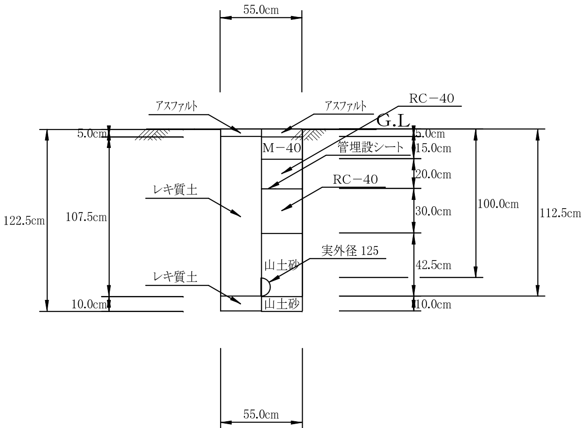
00:配水管 04: HPPE φ 100上水単独 (L) (H=1000) (掘削・埋戻し) 1／25
