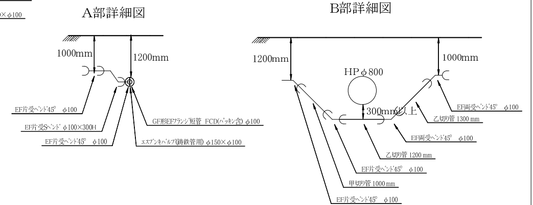
消火栓詳細図 S=1/20
