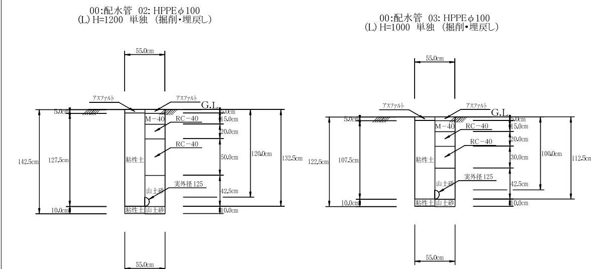
土工断面图 S=1/25
