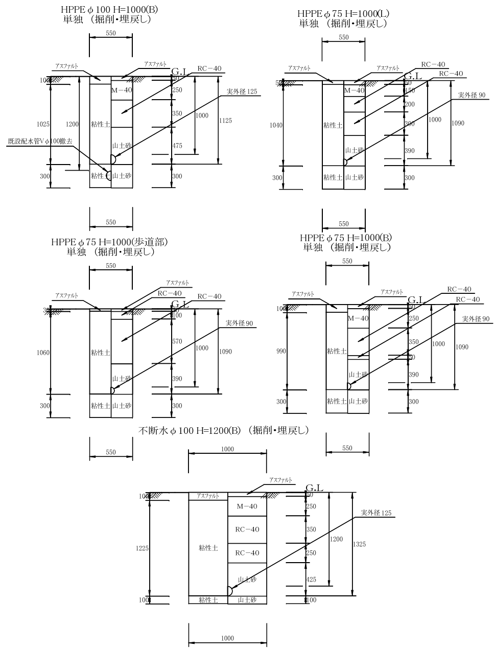
土工断面図 S=1/25
