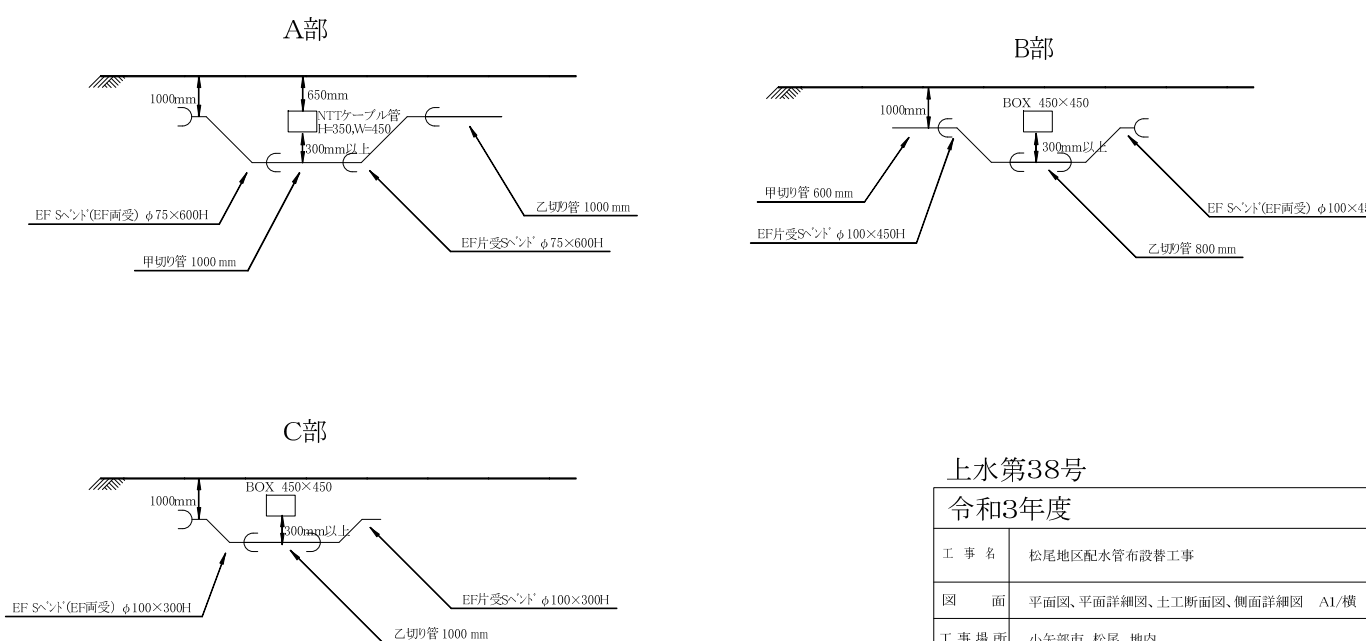
側面詳細図 S=1/100
