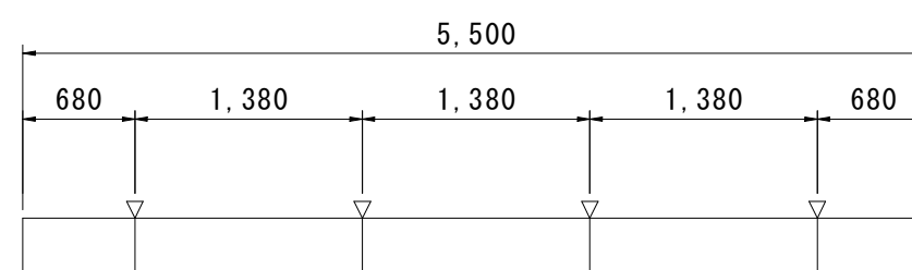
散水用ノズル位置
