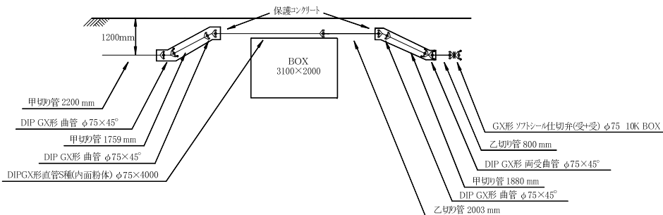
A部側面詳細図 1/100
