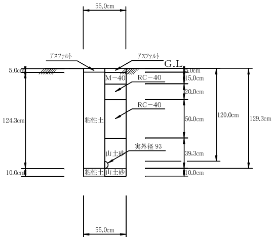
A部側面詳細図 1/100
