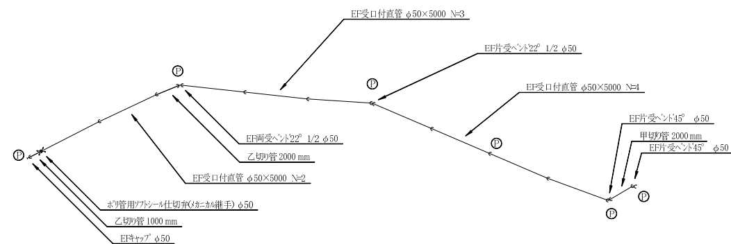
配管平面詳細図 S=1/200
