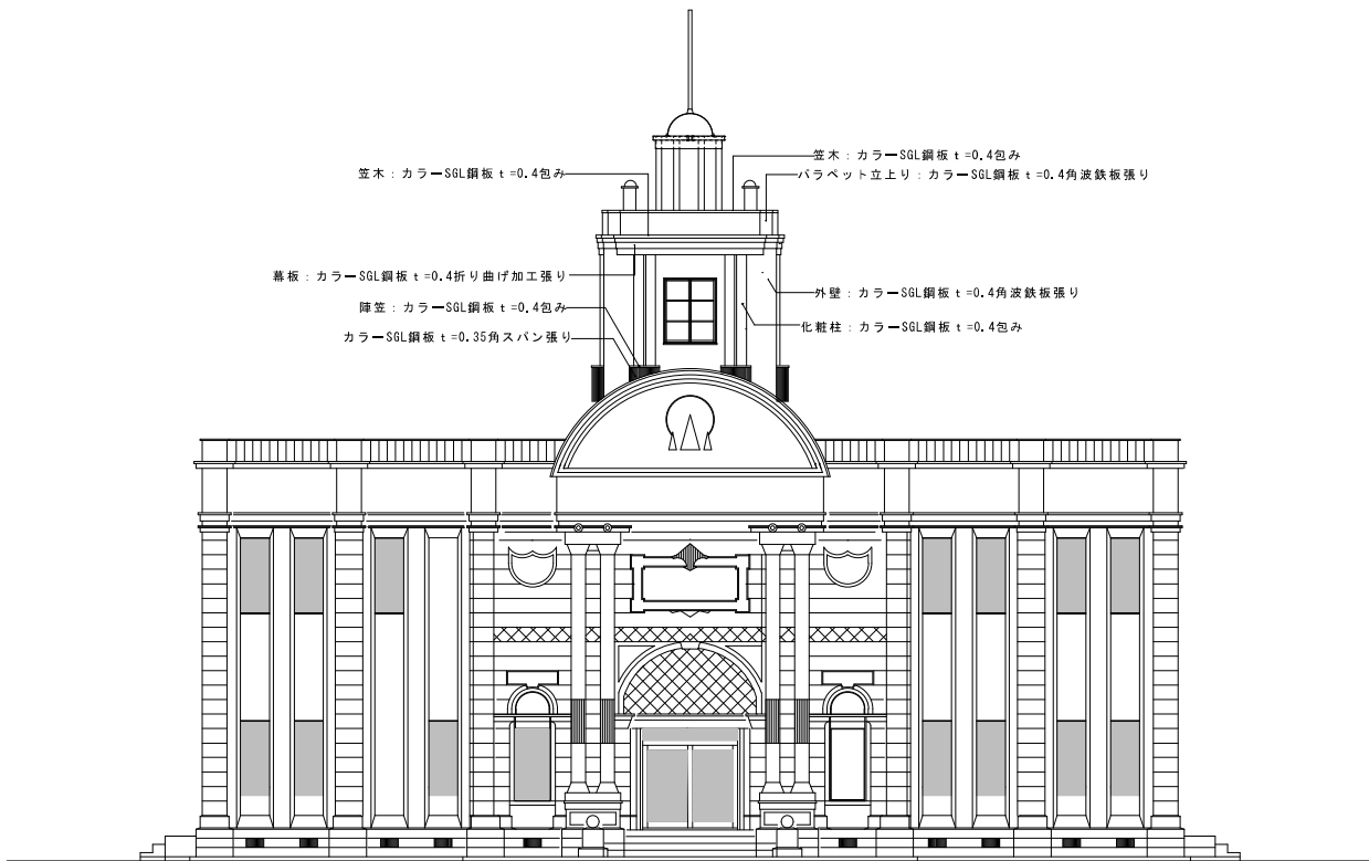
東側立面図
