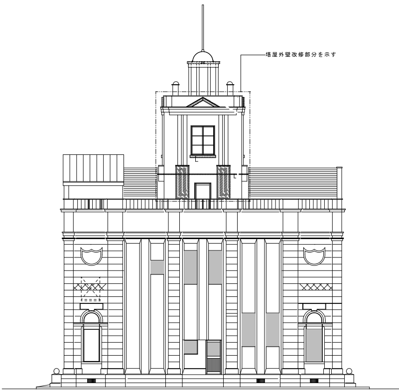
南側立面図
