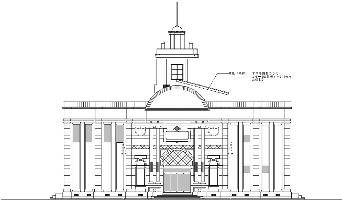
西側立面図
