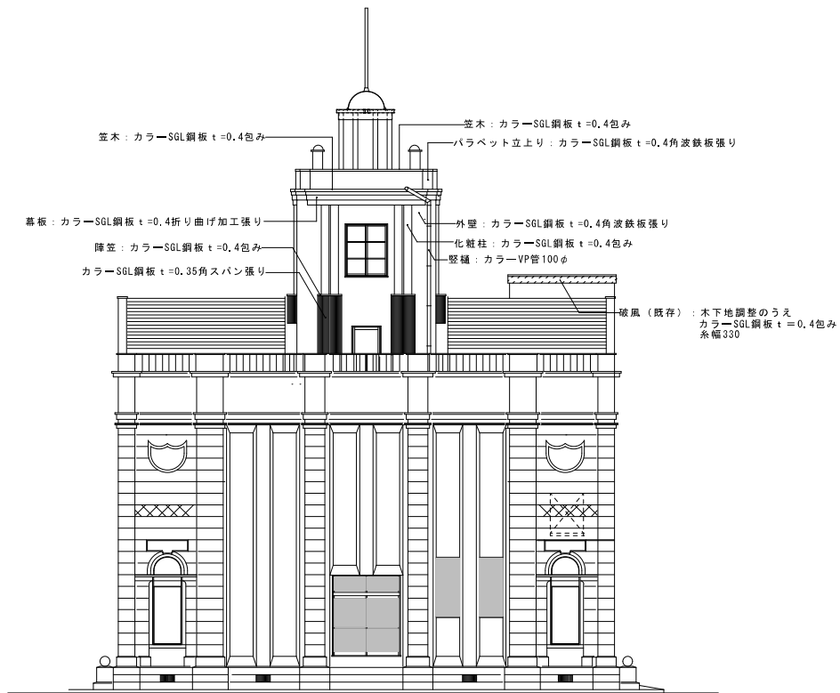
北側立面図
