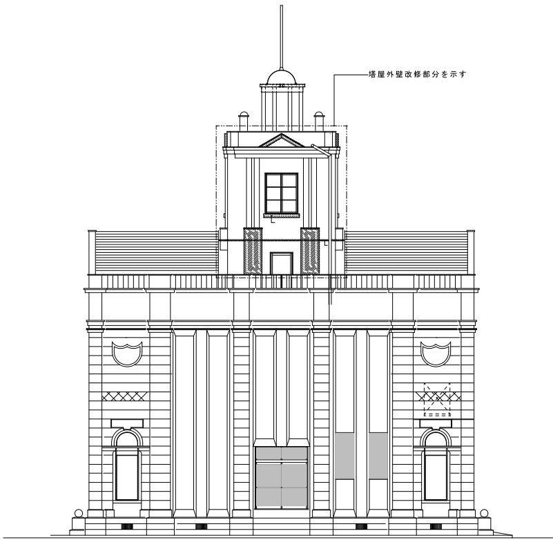
北側立面図
