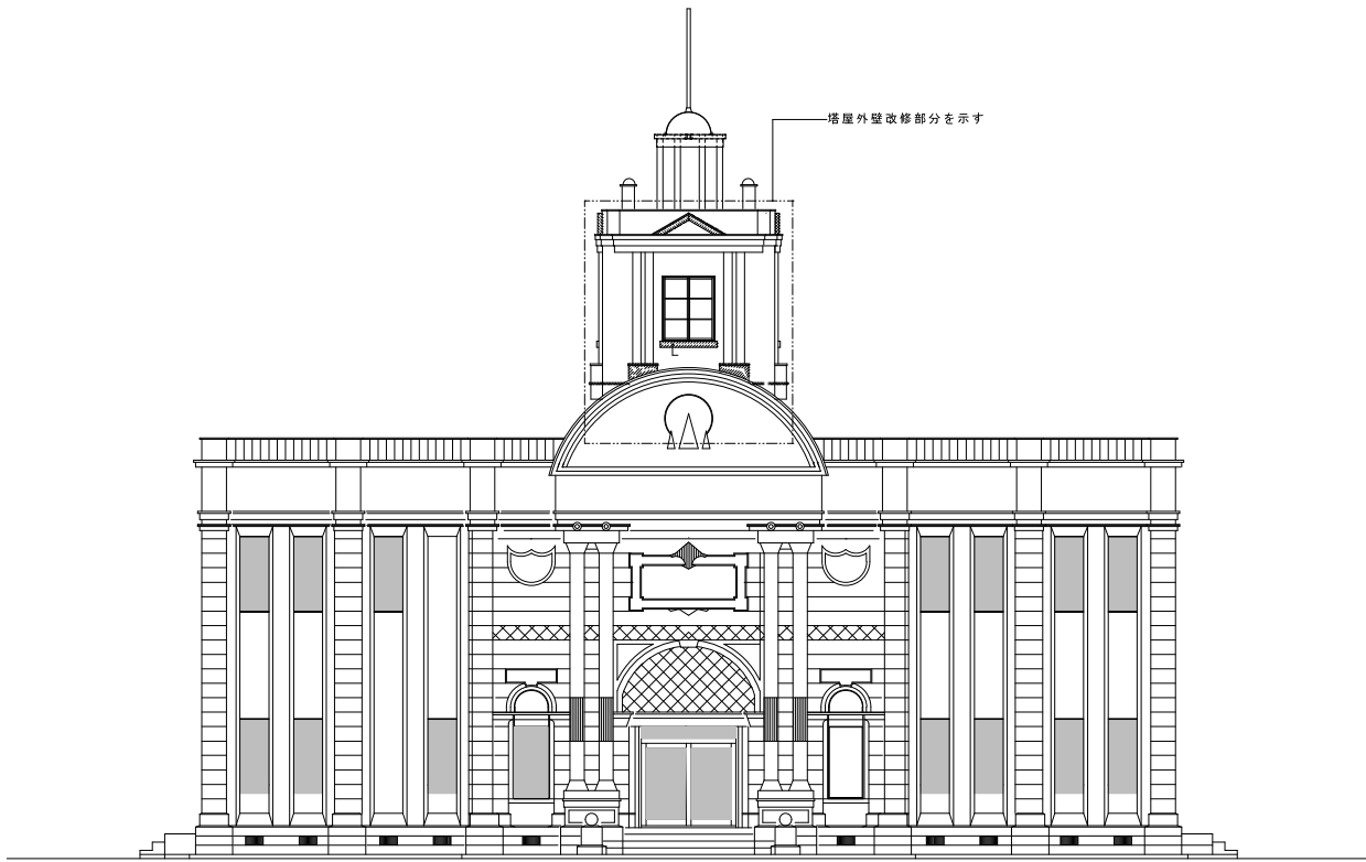
東側立面図
