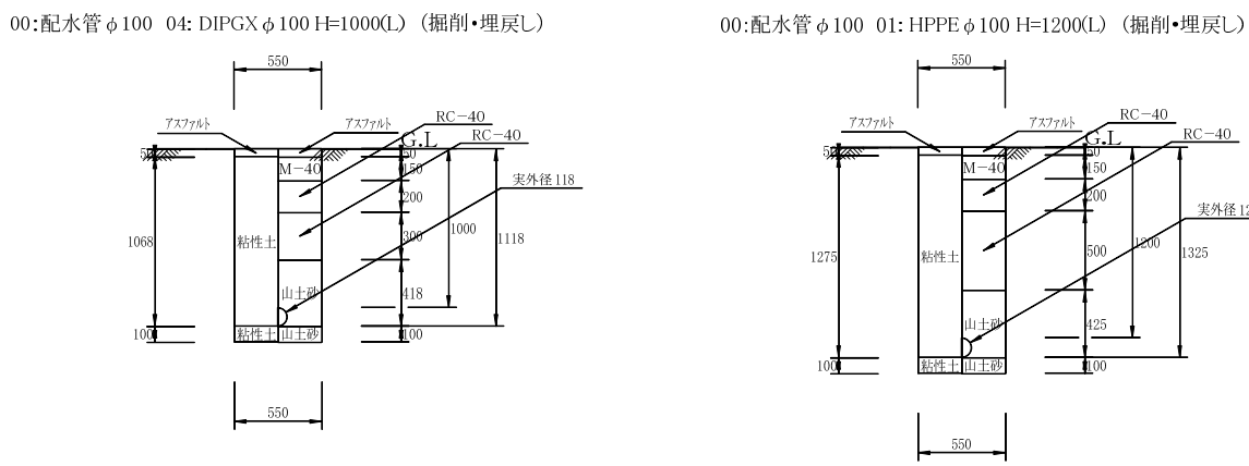
土工断面図 S=1/25
