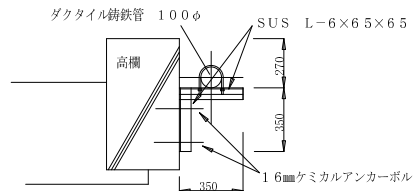
取付詳細図 1/20
