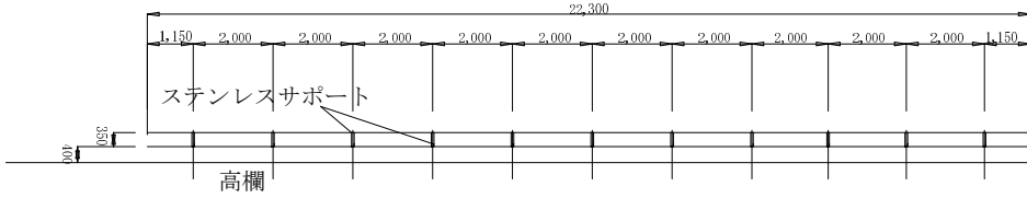
取付詳細図 1/20
