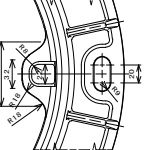
コネクタ受け部詳細図
