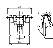
⑤ シールロック詳細図
