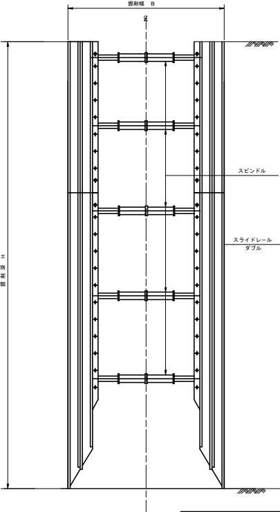
断面図
