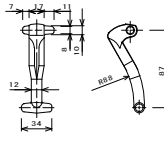
③ コネクタ詳細図
