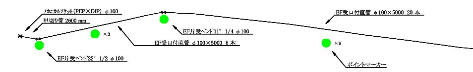
配管詳細平面図 S=1:200
