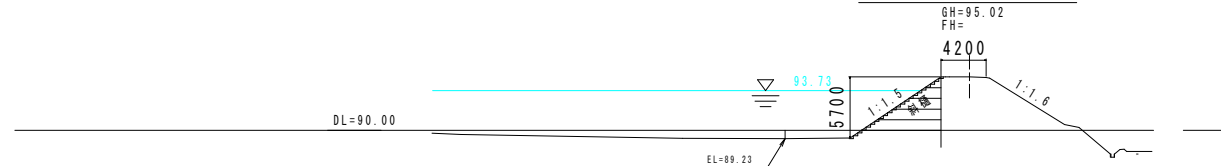
深淺測量1 s=1:500
