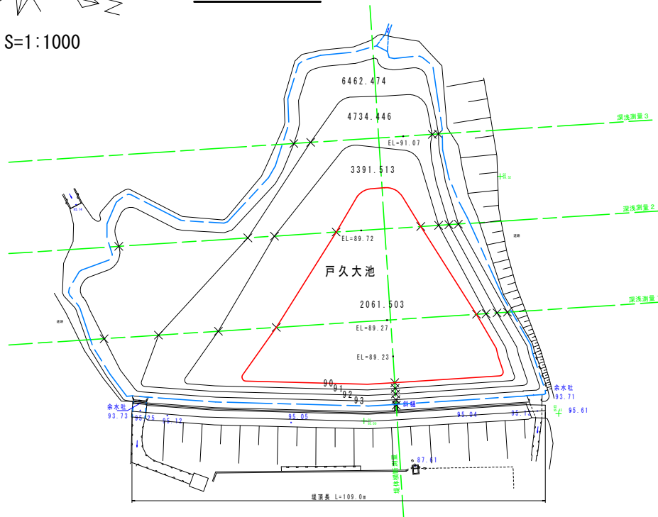
平面図 s=1:1000
