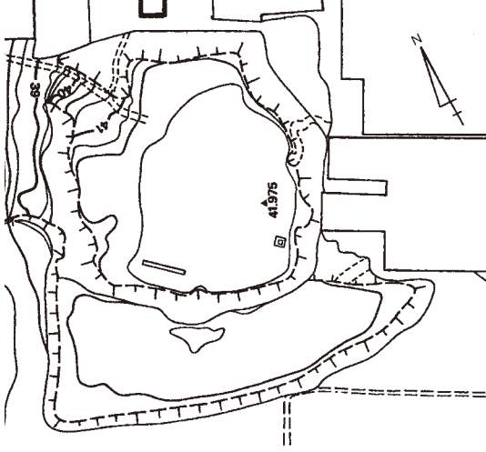
◀野端將軍塚古墳の平面図
