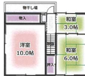
2階 縮尺 1/200
