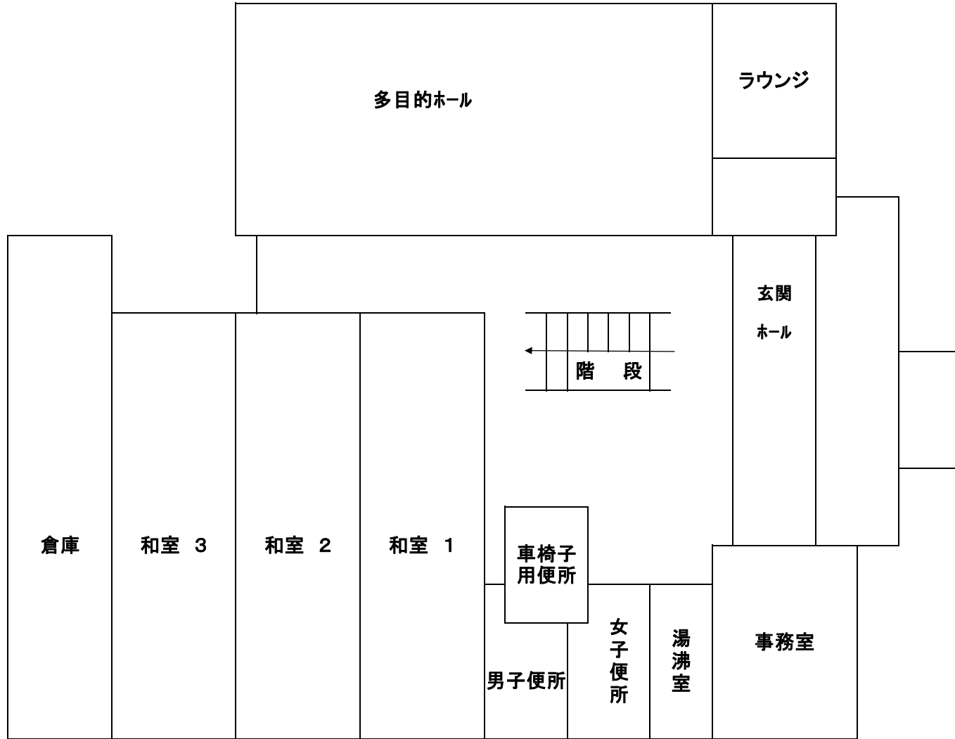
1階 平面図
